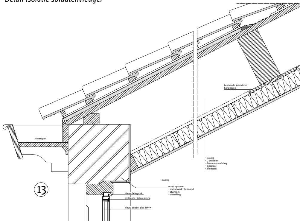
Detail isolatie soldatenvleugel
