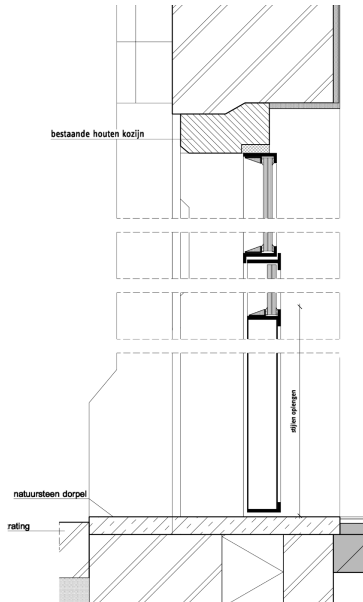
Detail stopverfprofilering deuren in gevels in kas
