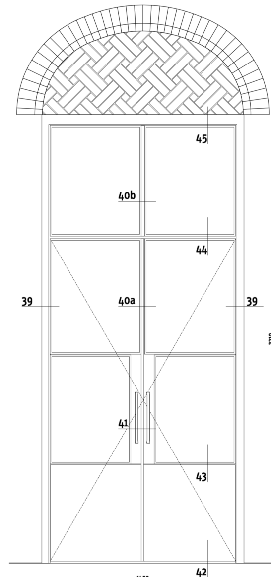
Aanzicht nieuwe deuren in gevels in kas
