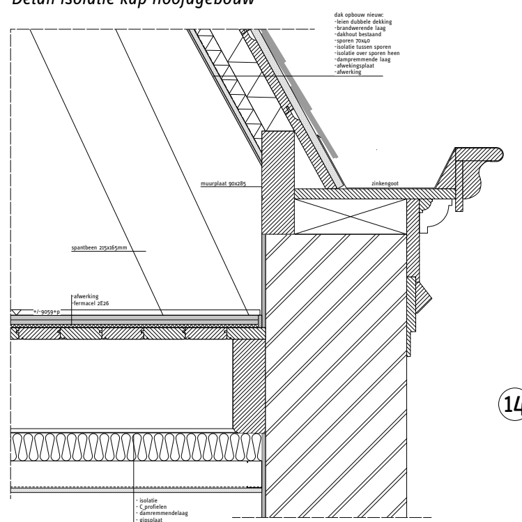
Detail isolatie kap hoofdgebouw
