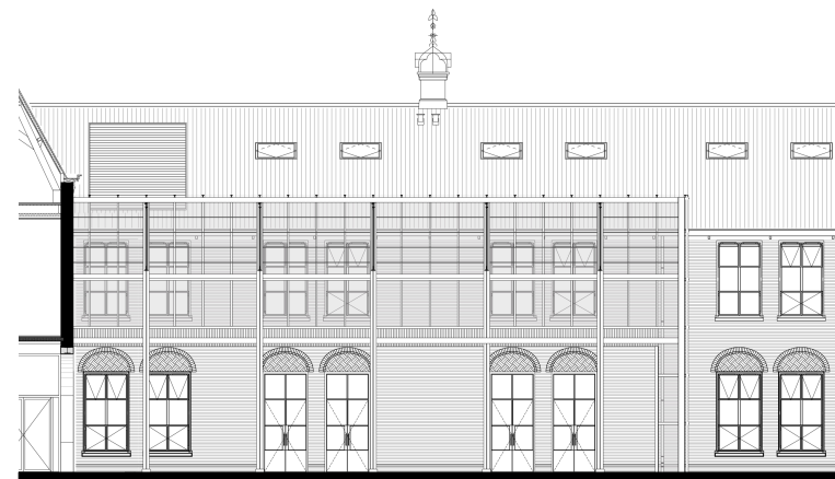
Langsdoorsnede met stramien uitgelijnd op kazernevleugel
