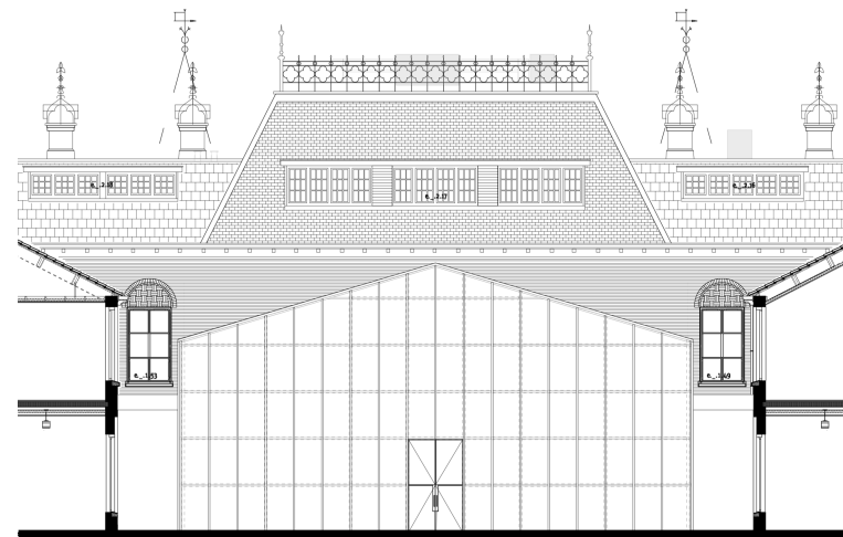
Kopgevel met verfijndere glas-indeling
