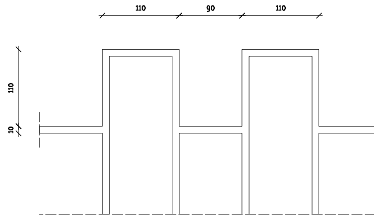
aanzicht detail balustrade
