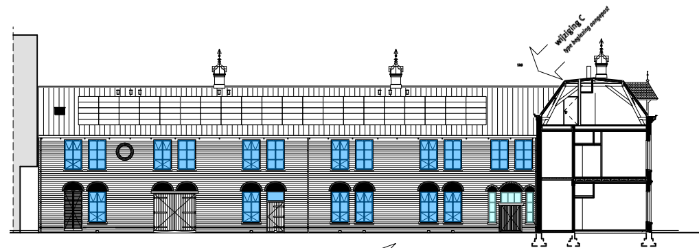
noordgevel vleugel B
