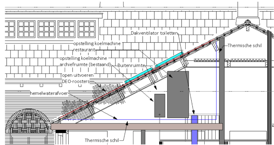
Principe-opstelling koelmachines in installatiezone
