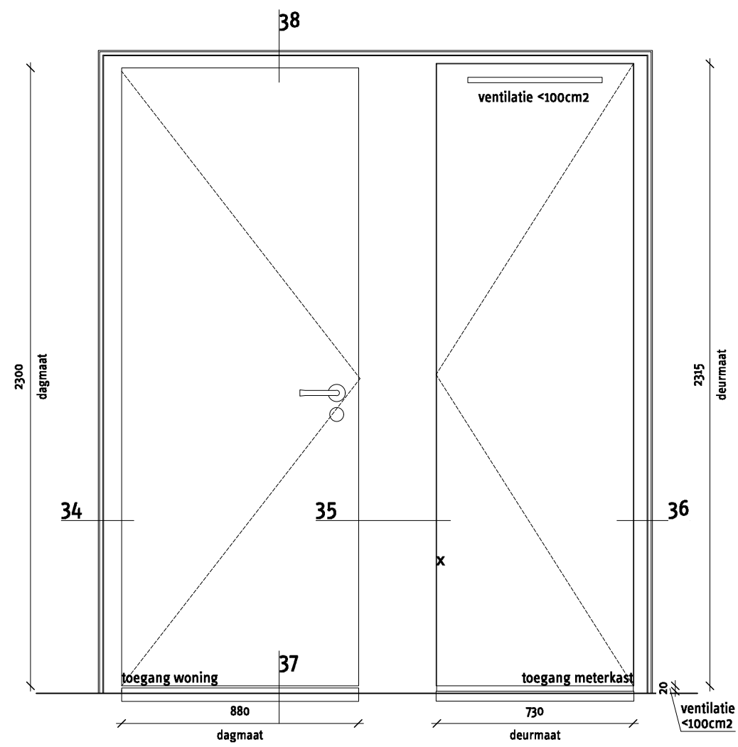
entree deur woningen met meterkastdeur. soldaten vleugels A/B/C/D
