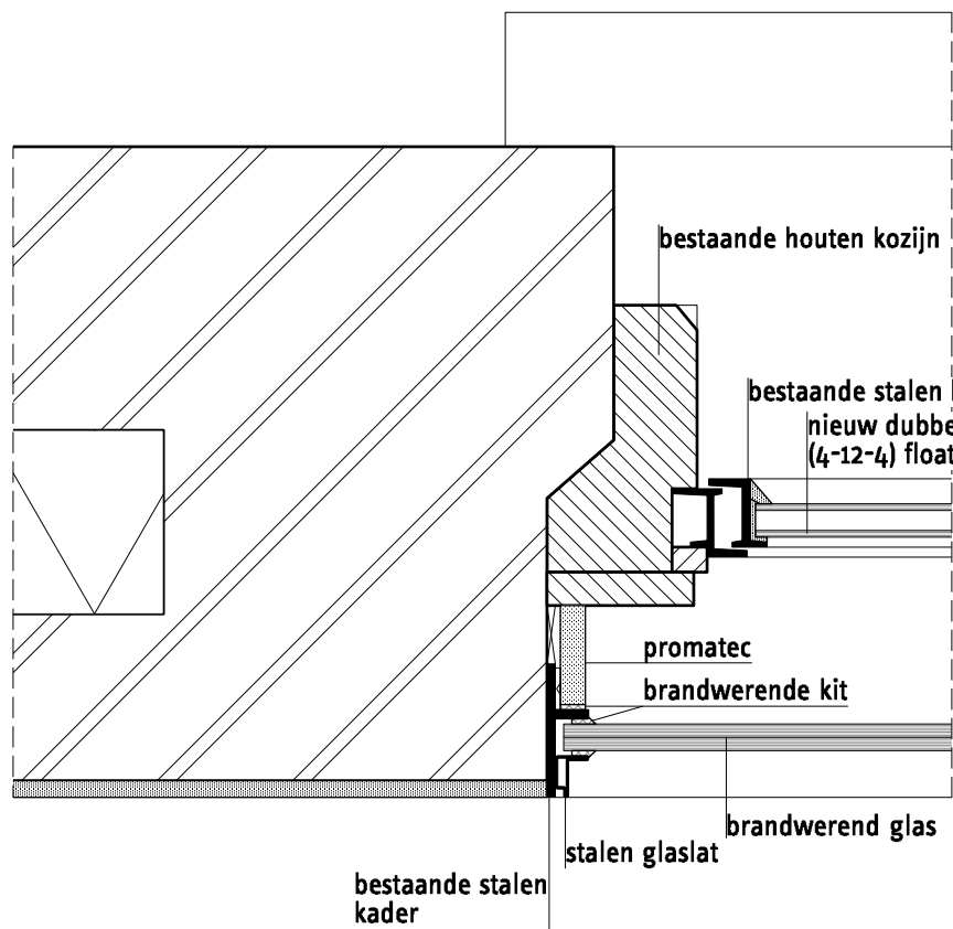
buiten zijde stalen kozijn met brandwerend achterzetaam openbare ruimte
