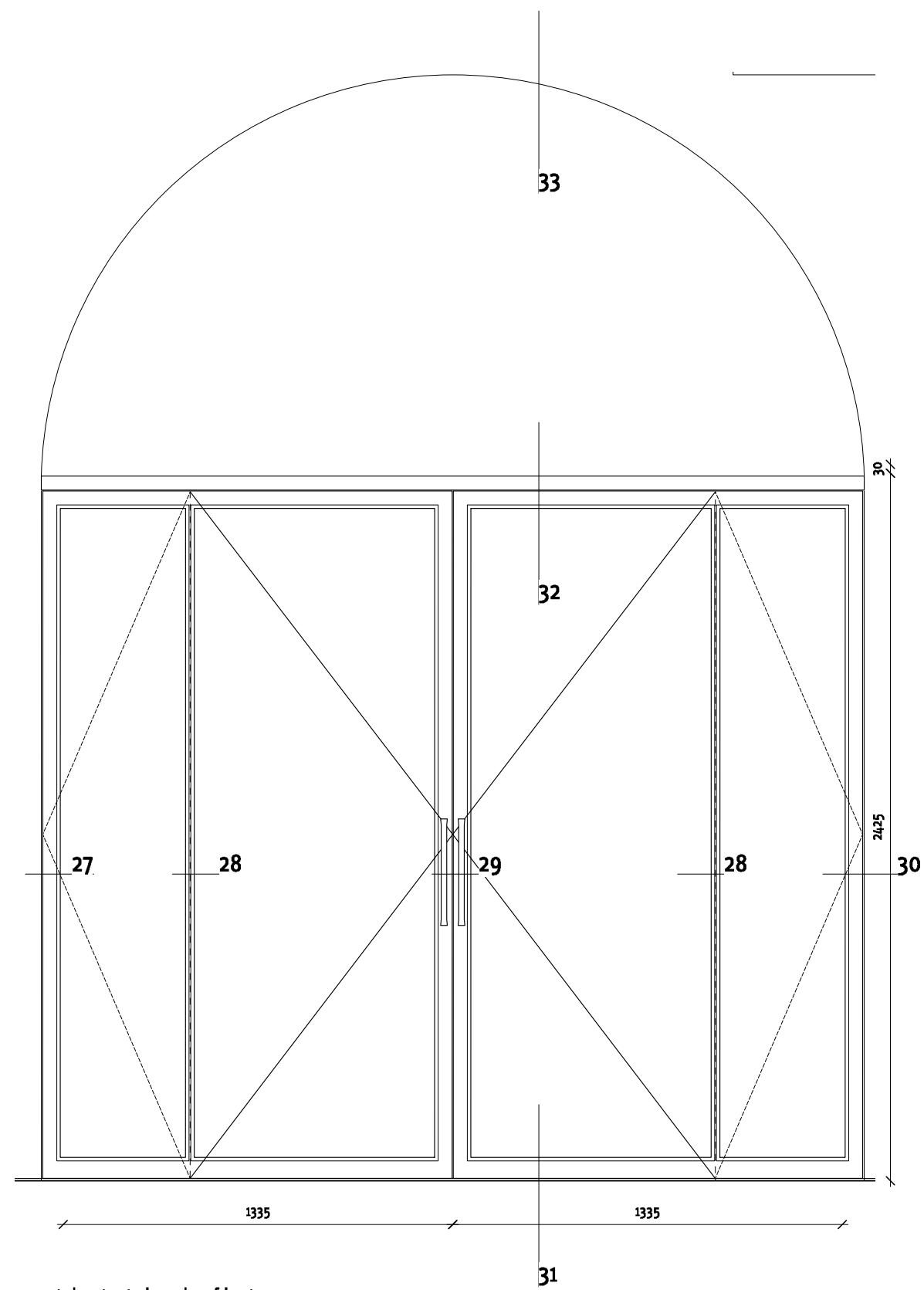
staal taatsdeur hoofdentree gezien van uit de gang.
