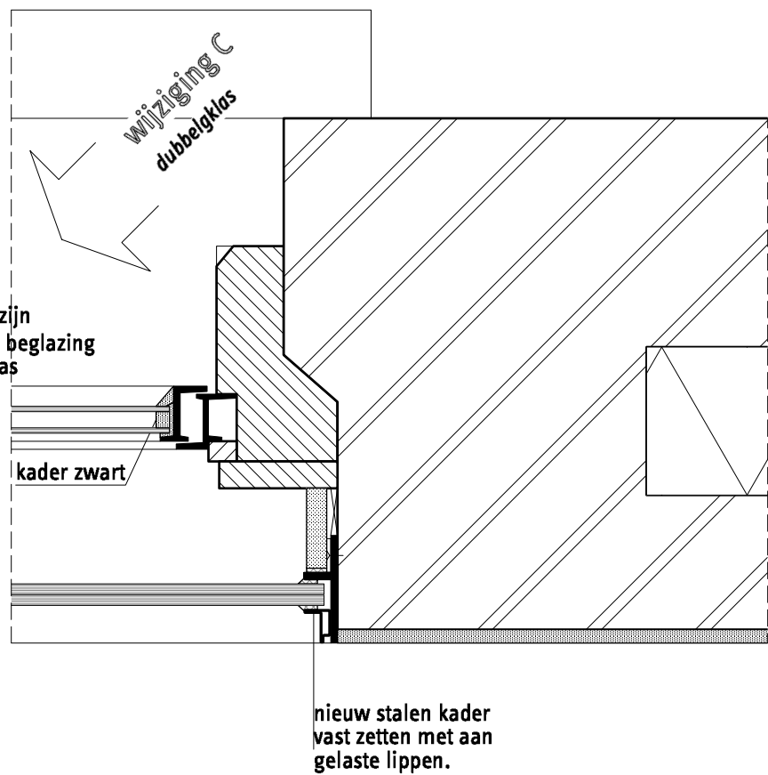
binnen zijde stalen kozijn met brandwerend achterzetaam openbare ruimte
