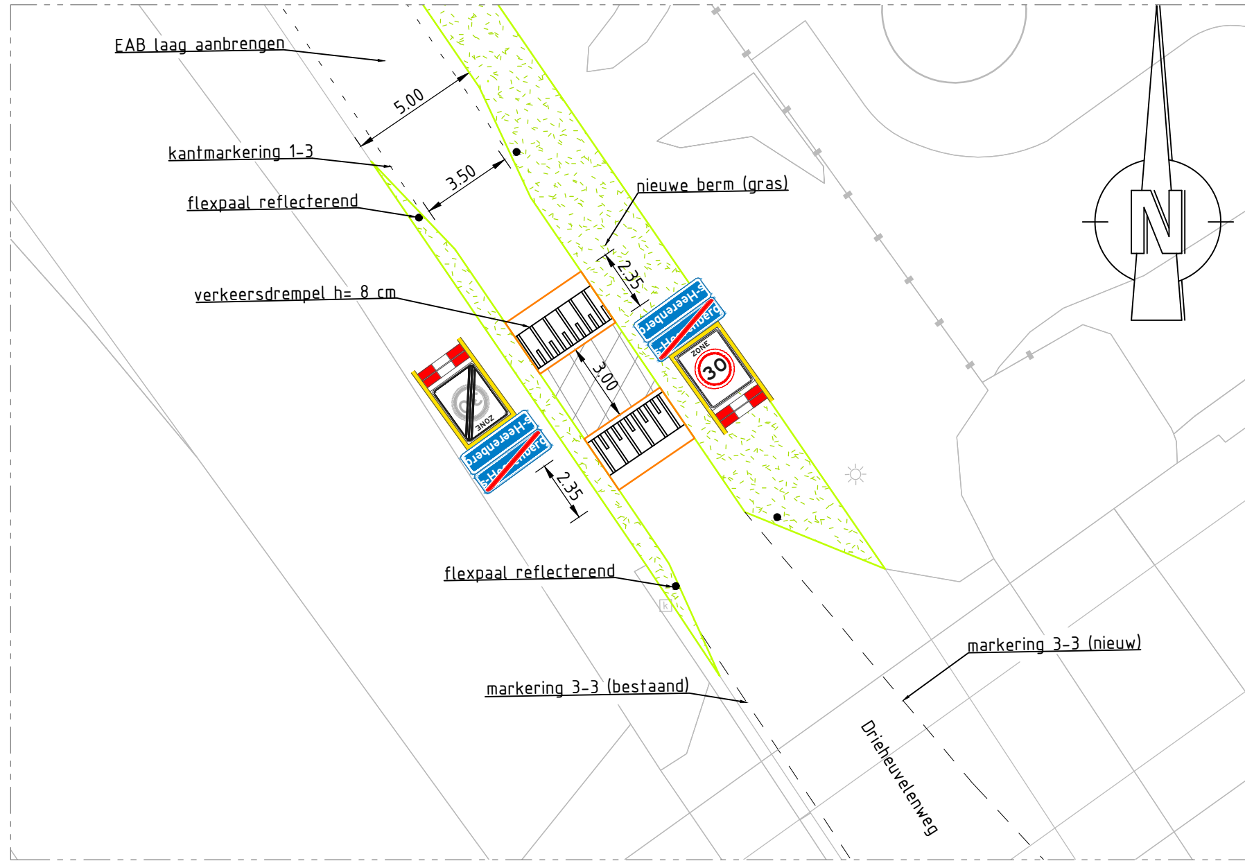
DETAIL 2 schaal 1:200
