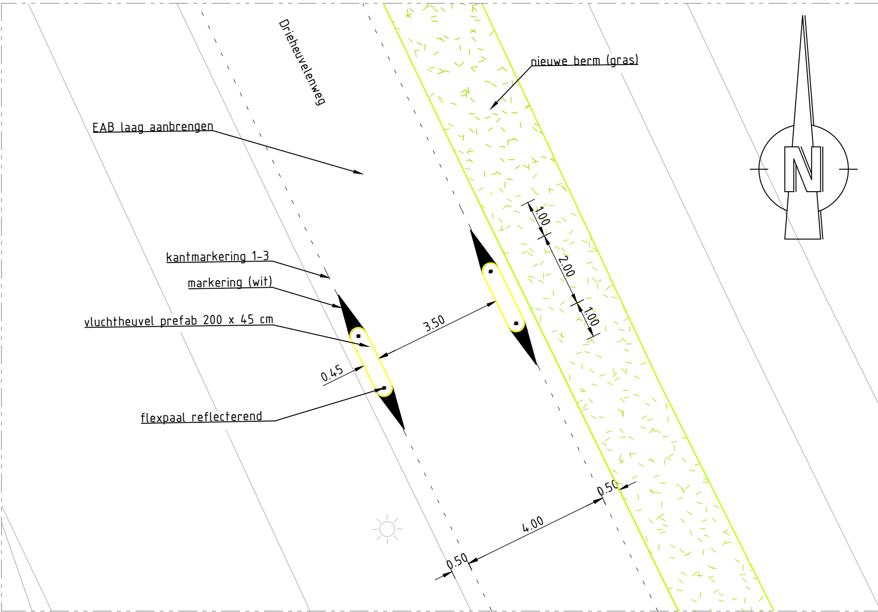
DETAIL 1 schaal 1:100
