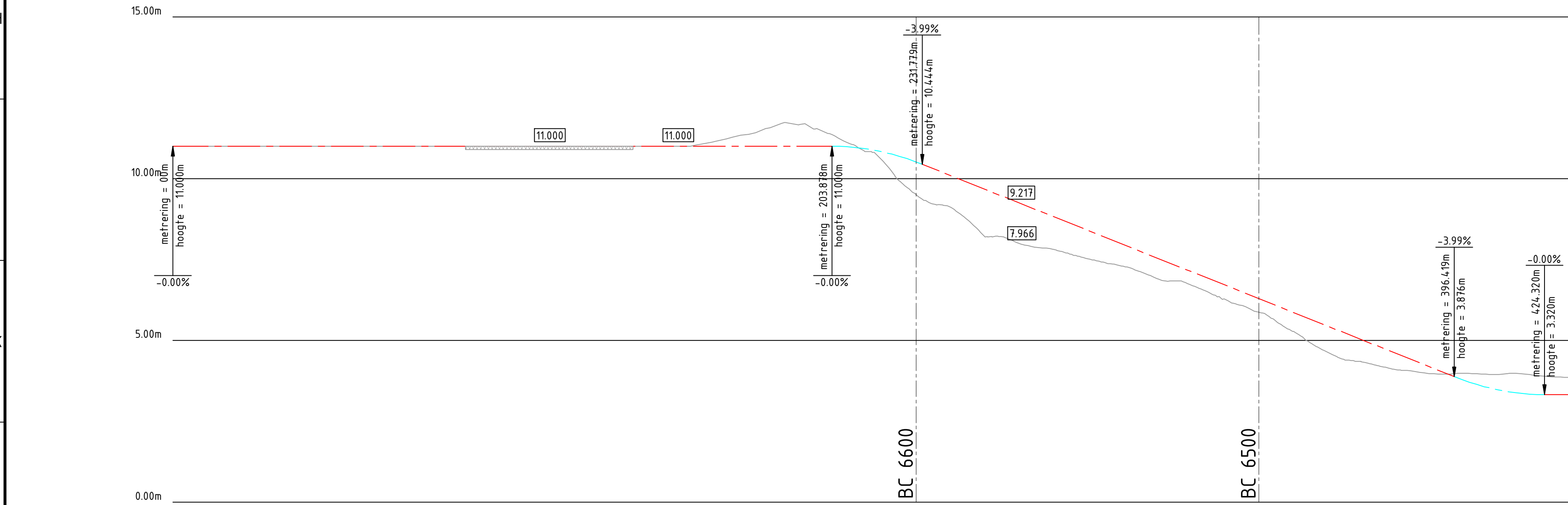
Lengteprofiel as ALM-Duindoorssteek 3 (P5) Metrering 0.000 tot 431.517
