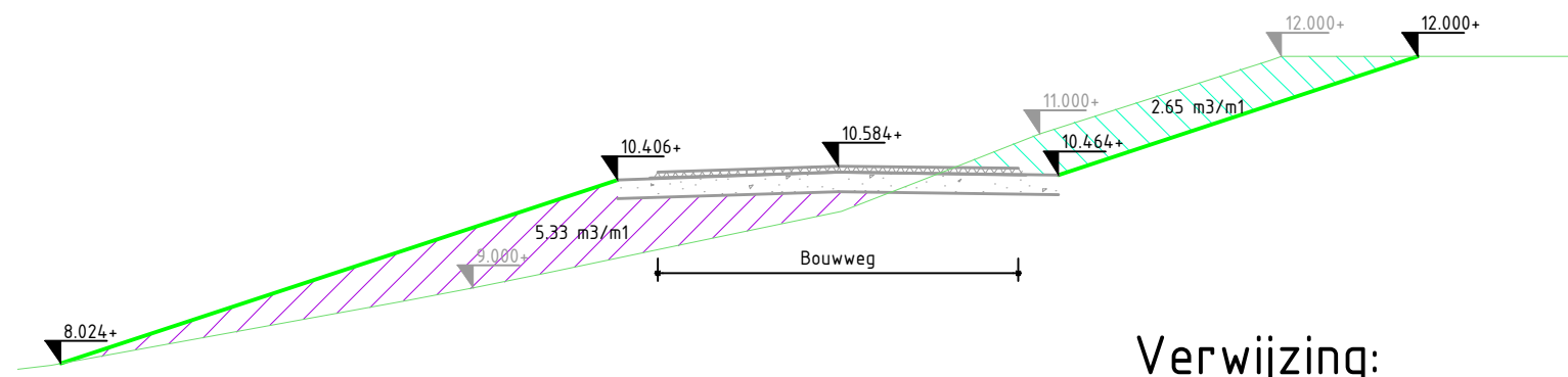
Dwarsprofiel BC 6600 Schaal 1:100
