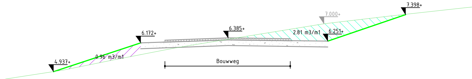
Dwarsprofiel BC 6500 Schaal 1:100
