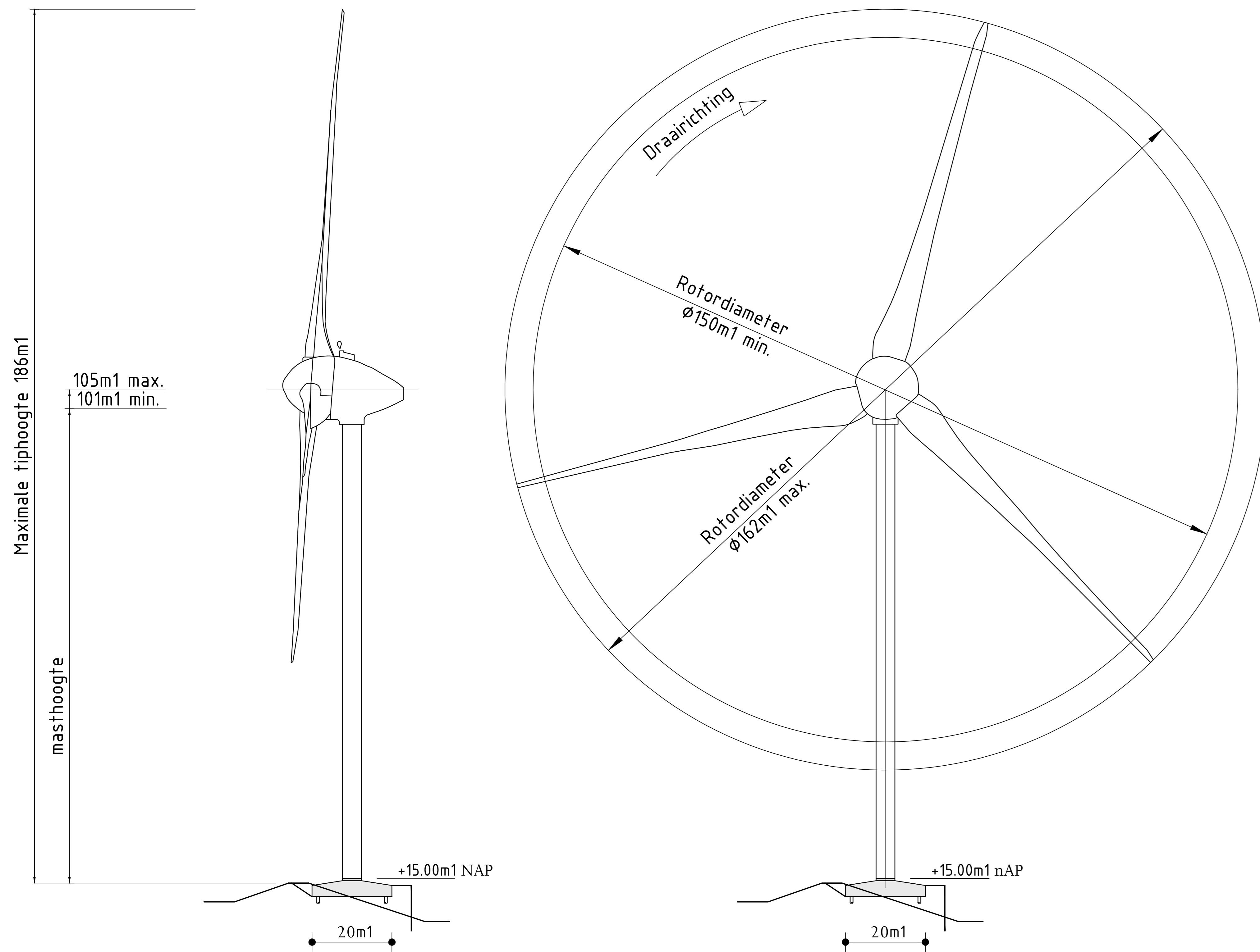
Windturbine Maasvlakte 2
