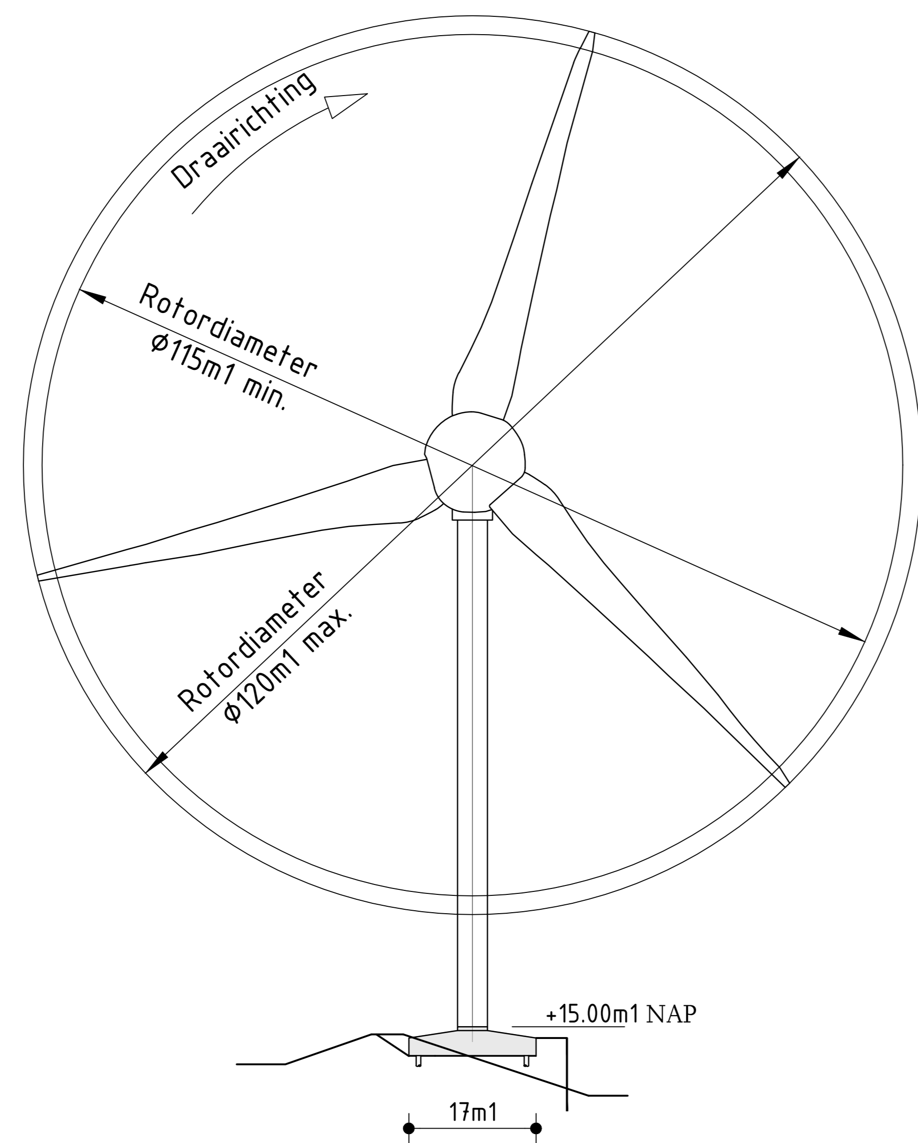
Windturbine Maasvlakte 2
