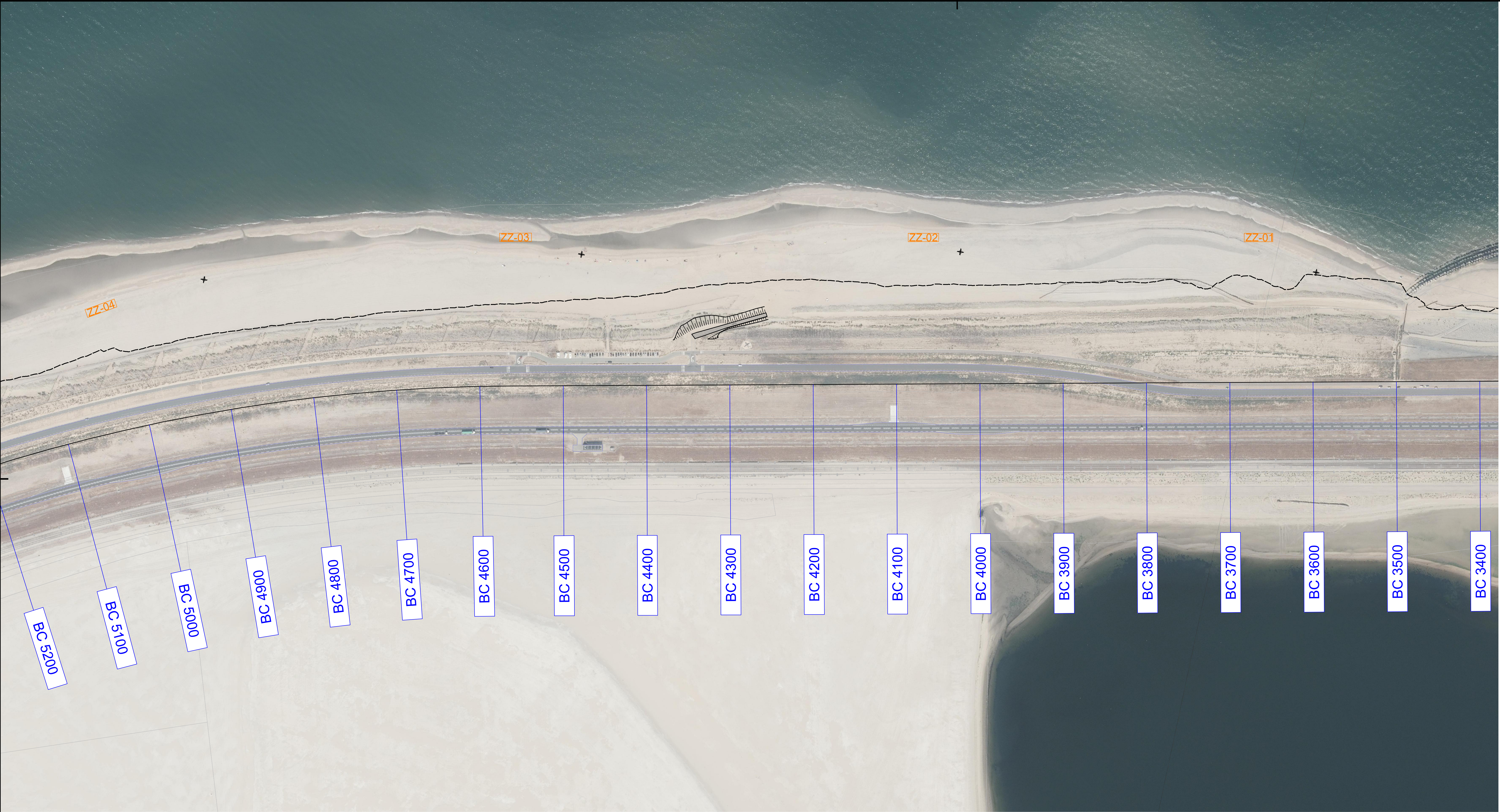
Overzicht Schaal 1:2000
