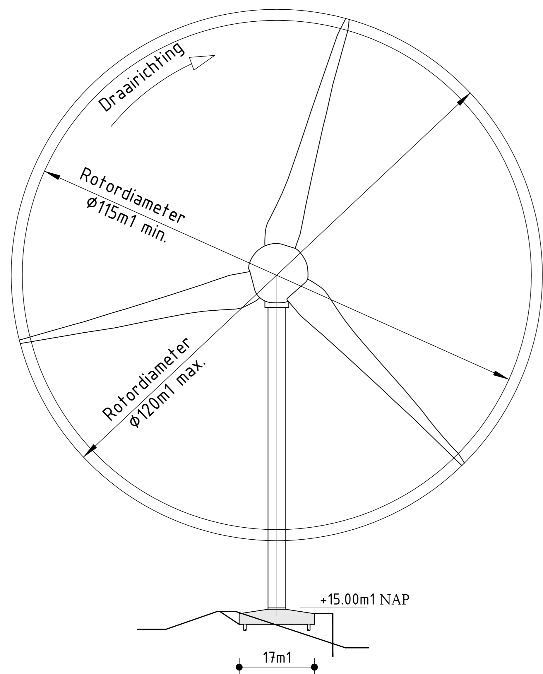
Windturbine Maasvlakte 2
