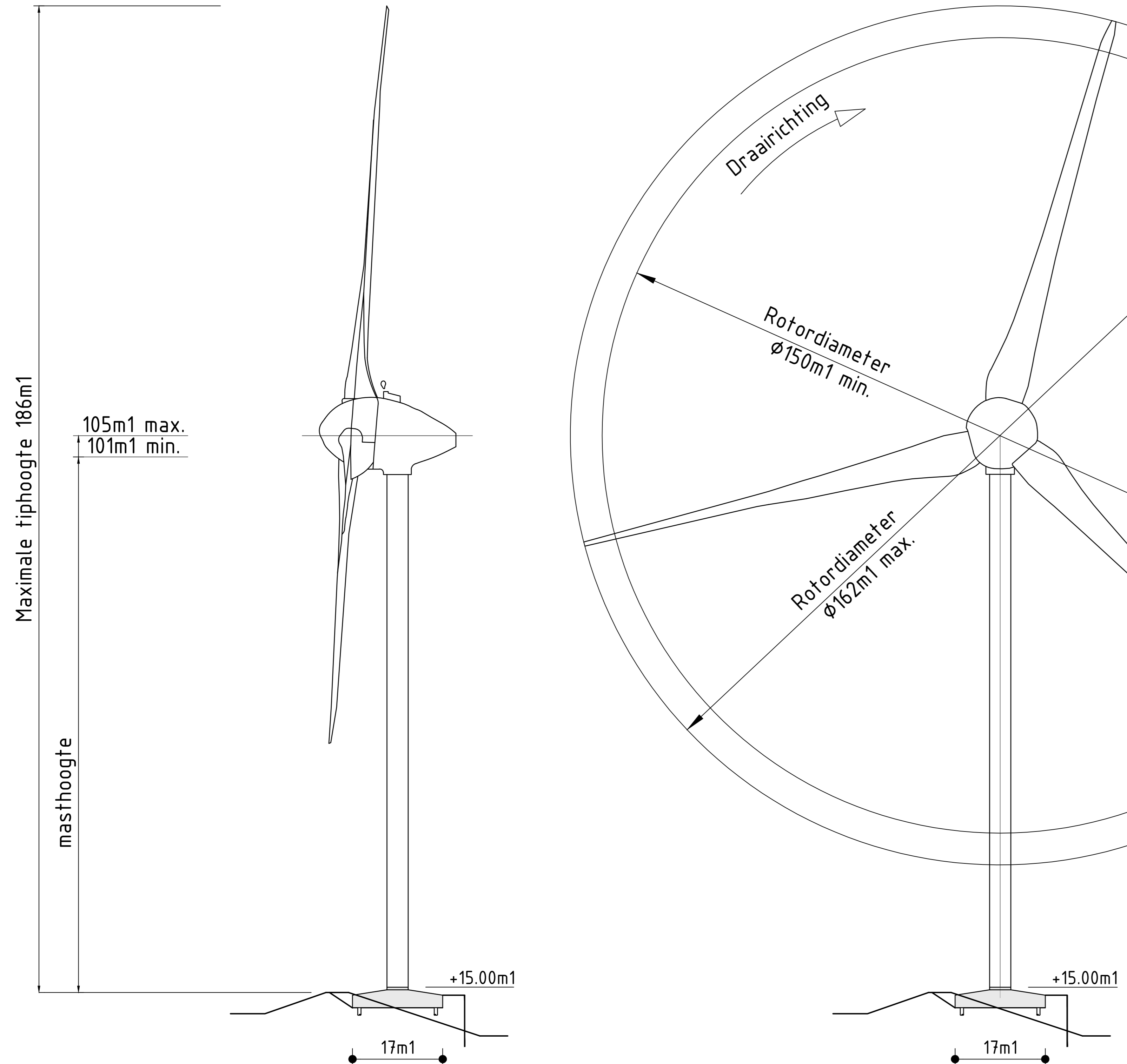
Windturbine Maasvlakte 2
