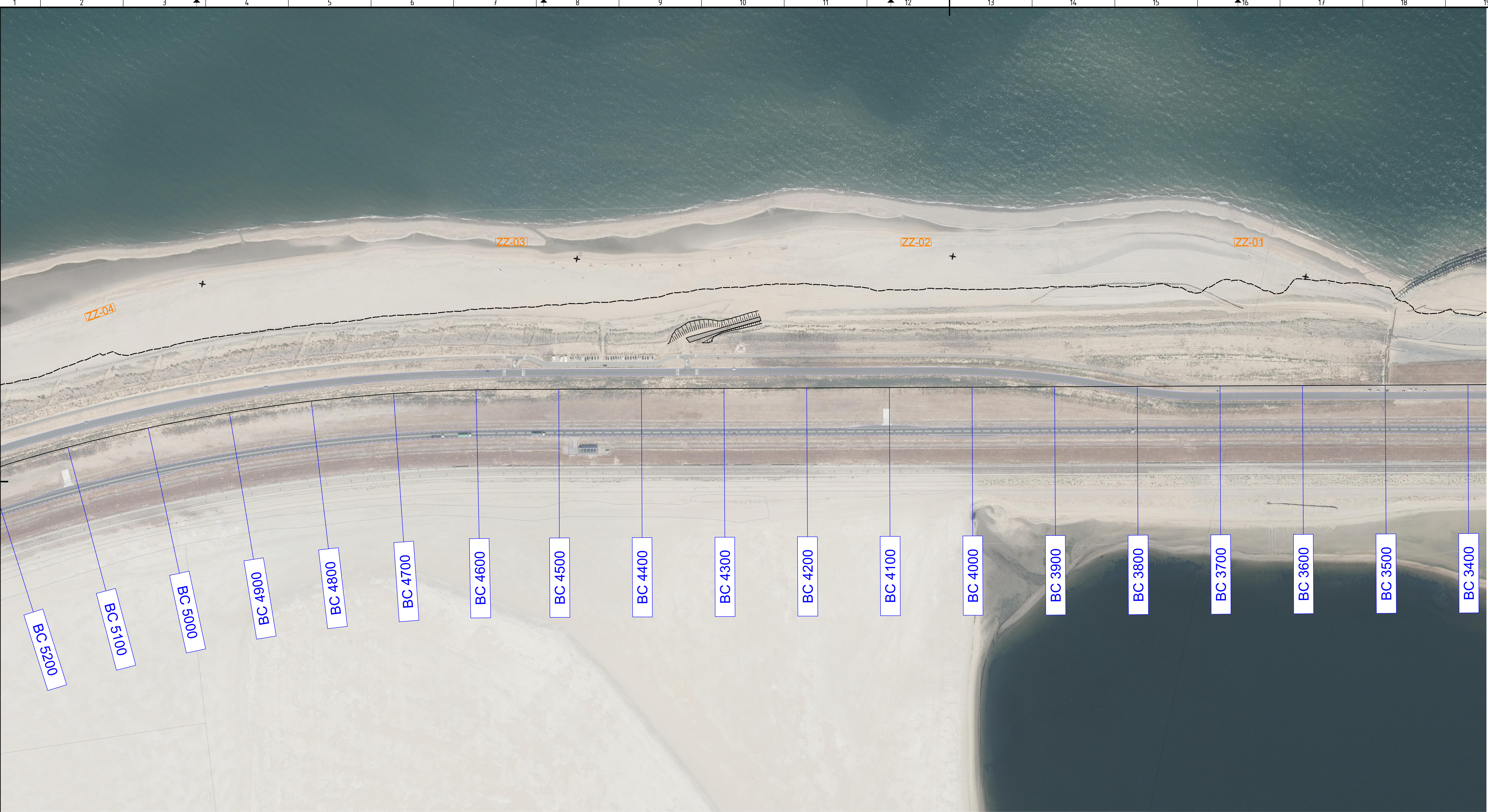
Overzicht Schaal 1:2000
