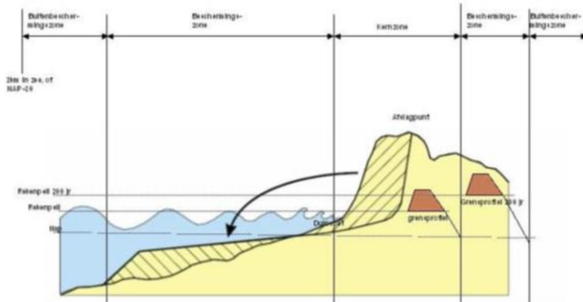
AFBEELDING 20.6 GRENSPROFIEL ZEEWERING
