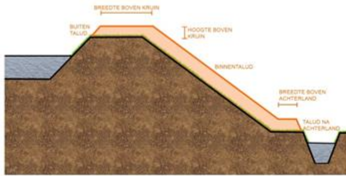
leggerprofiel (zwarte lijn) en profiel van vrije ruimte (oranje lijn)
