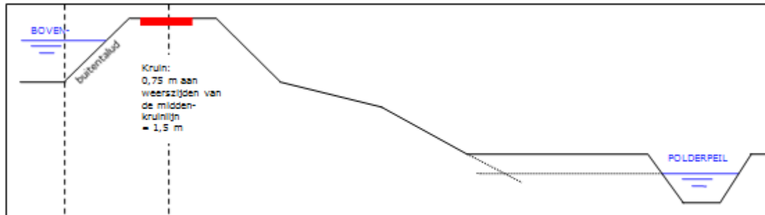
AFBEELDING 20.3 KRUIJN VAN DE WATERKERING
