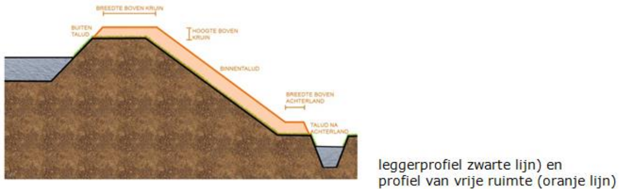
AFBEELDING 25.4 PROFIEL VAN VRIJE RUIMTE (ORANJE LIJN)
