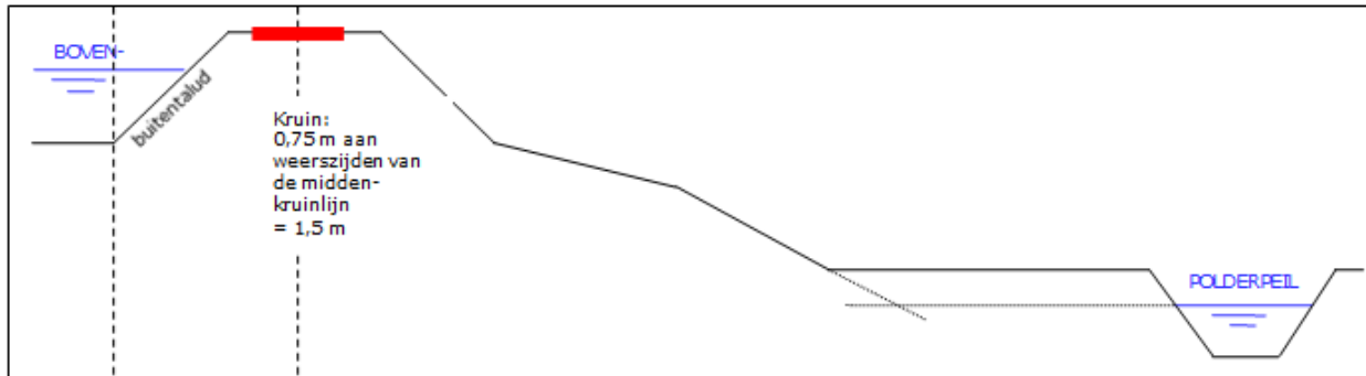
AFBEELDING 19.3 LIGGING VAN DE KRUIJN VAN DE WATERKERING
