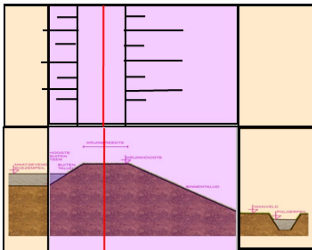
AFBEELDING 21.2 OVERZICHT LEGGERZONES WATERKERINGEN
