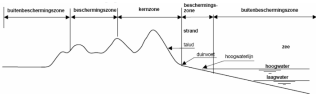
AFBEELDING 21.1 OVERZICHT LEGGERZONES ZEEWERING
