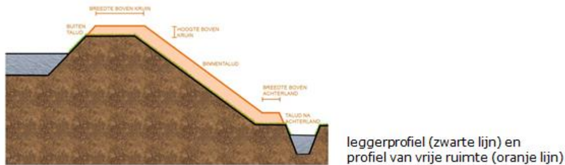
AFBEELDING 20.4 PROFIEL VAN VRIJE RUIMTE
