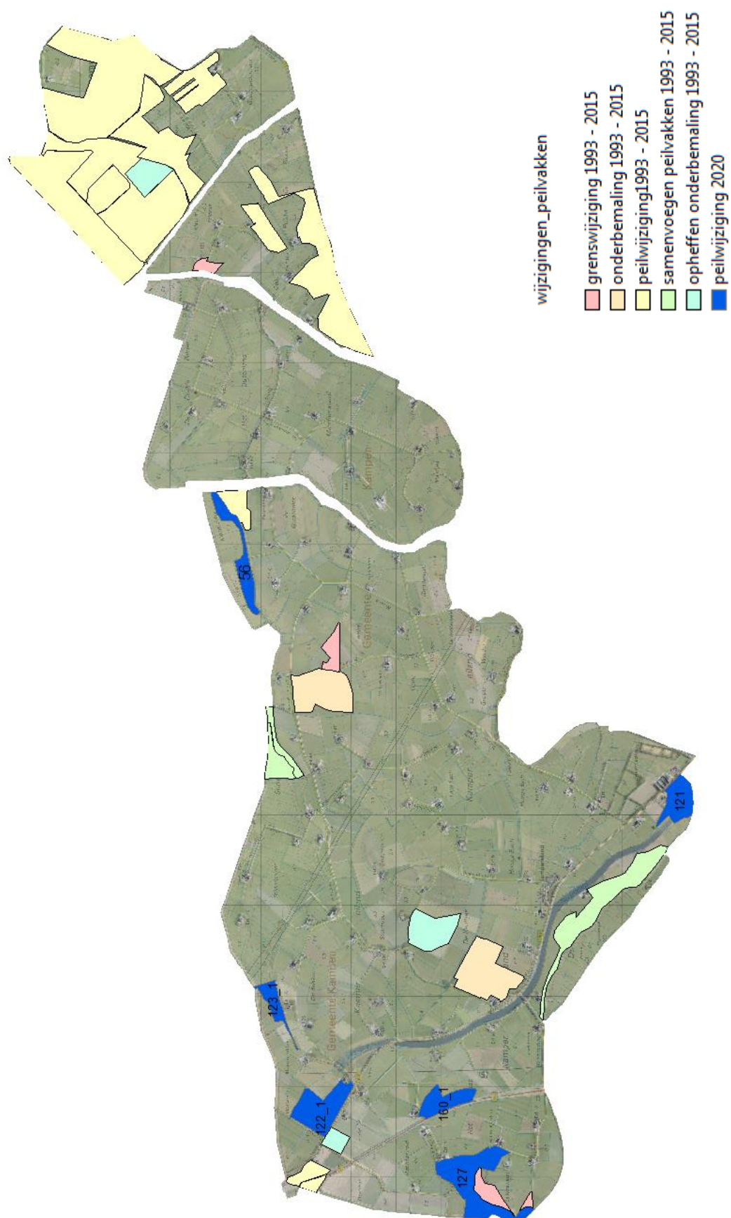
FIGUUR 14 PEILWIJZIGINGEN 1993 – 2015 EN PEILWIJZIGINGEN 2020 VOOR HET PEILBESLUIT KAMPEREILAND, MANDJESWAARD, DE PIEPER EN ZUIDERZEEPOLDER
