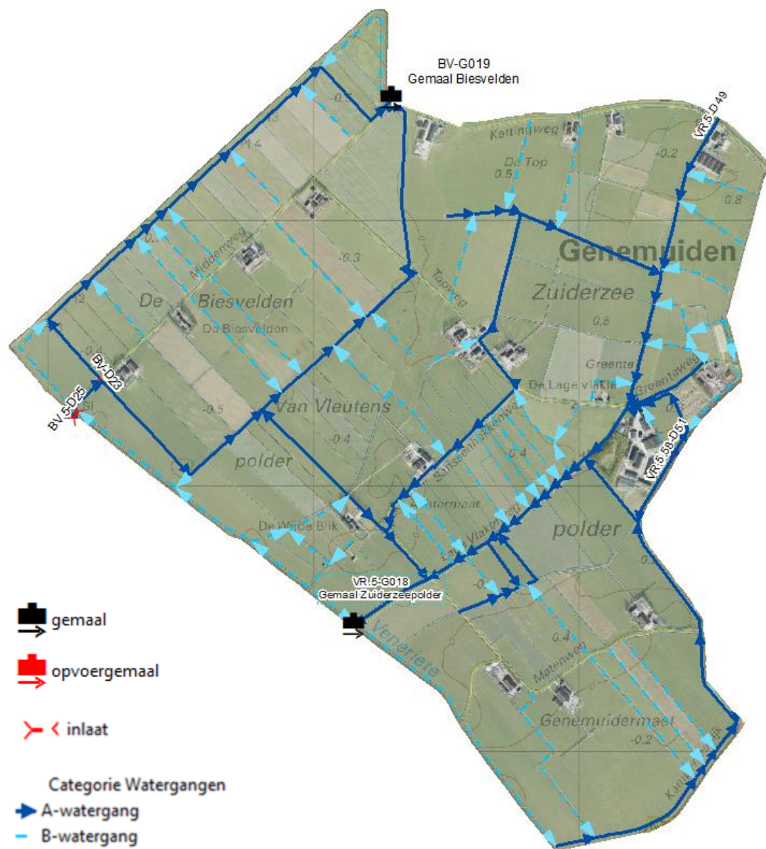
FIGUUR 5 OPPERVLAKTEWATERSYSTEEM ZUIDERZEEPOLDER EN POLDER DE BIESVELDEN
