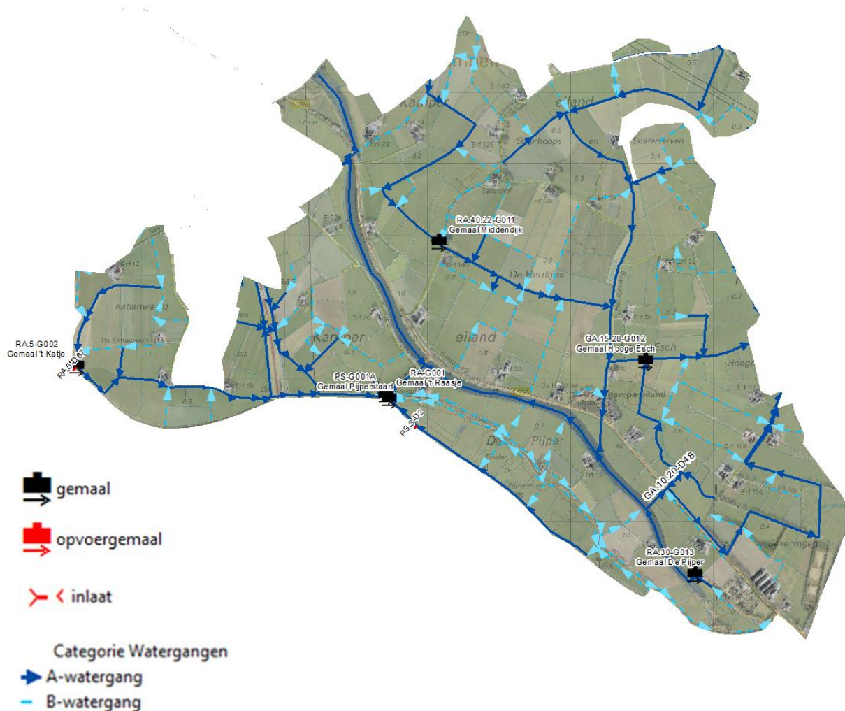
FIGUUR 11 OPPERVLAKTEWATERSYSTEEM 'T RAASJE EN PIJPERSTAART
