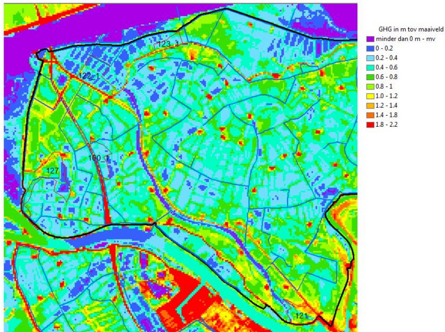
KAART 10 GEMIDDELD HOOGSTE GRONDWATERSTAND
