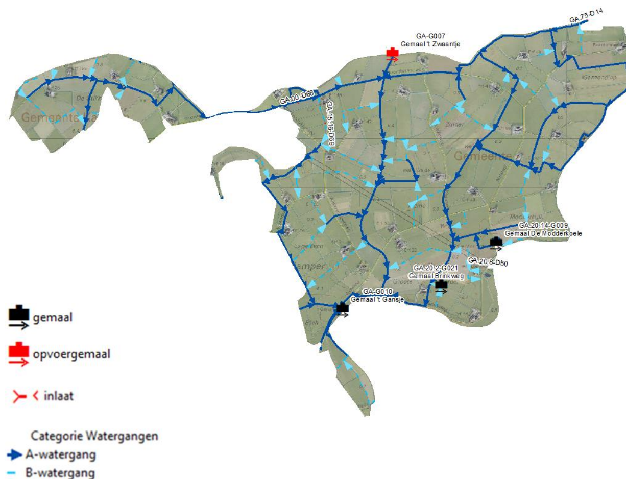
FIGUUR 12 OPPERVLAKTEWATERSYSTEEM POLDER 'T GANSJE
