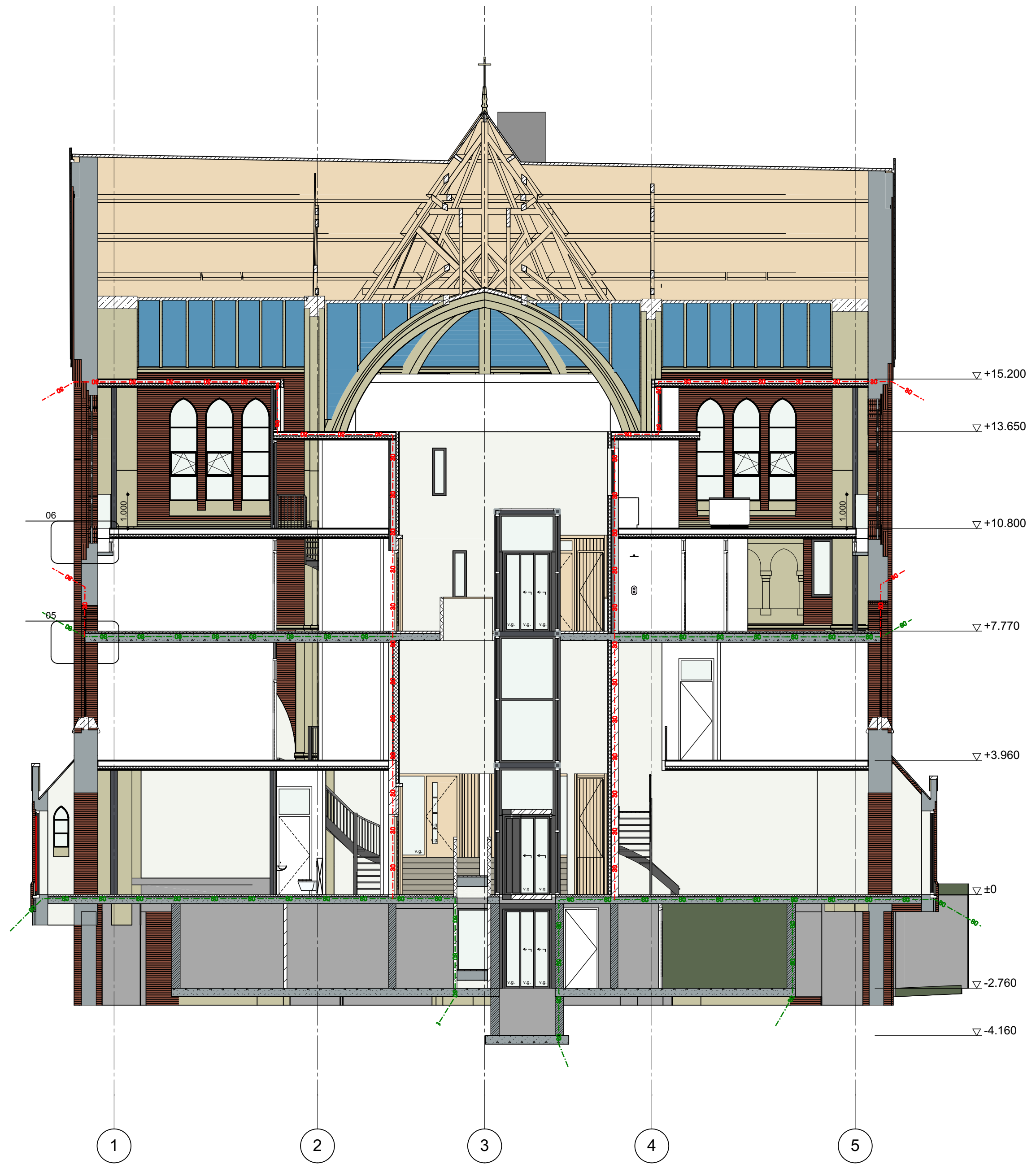
Doorsnede E-E
