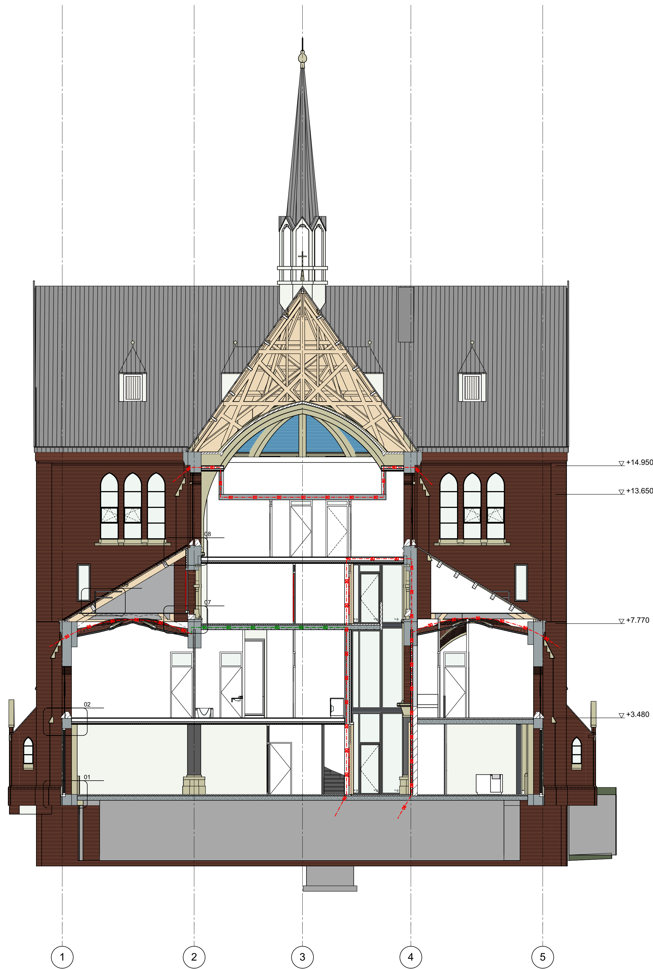
Doorsnede D-D
