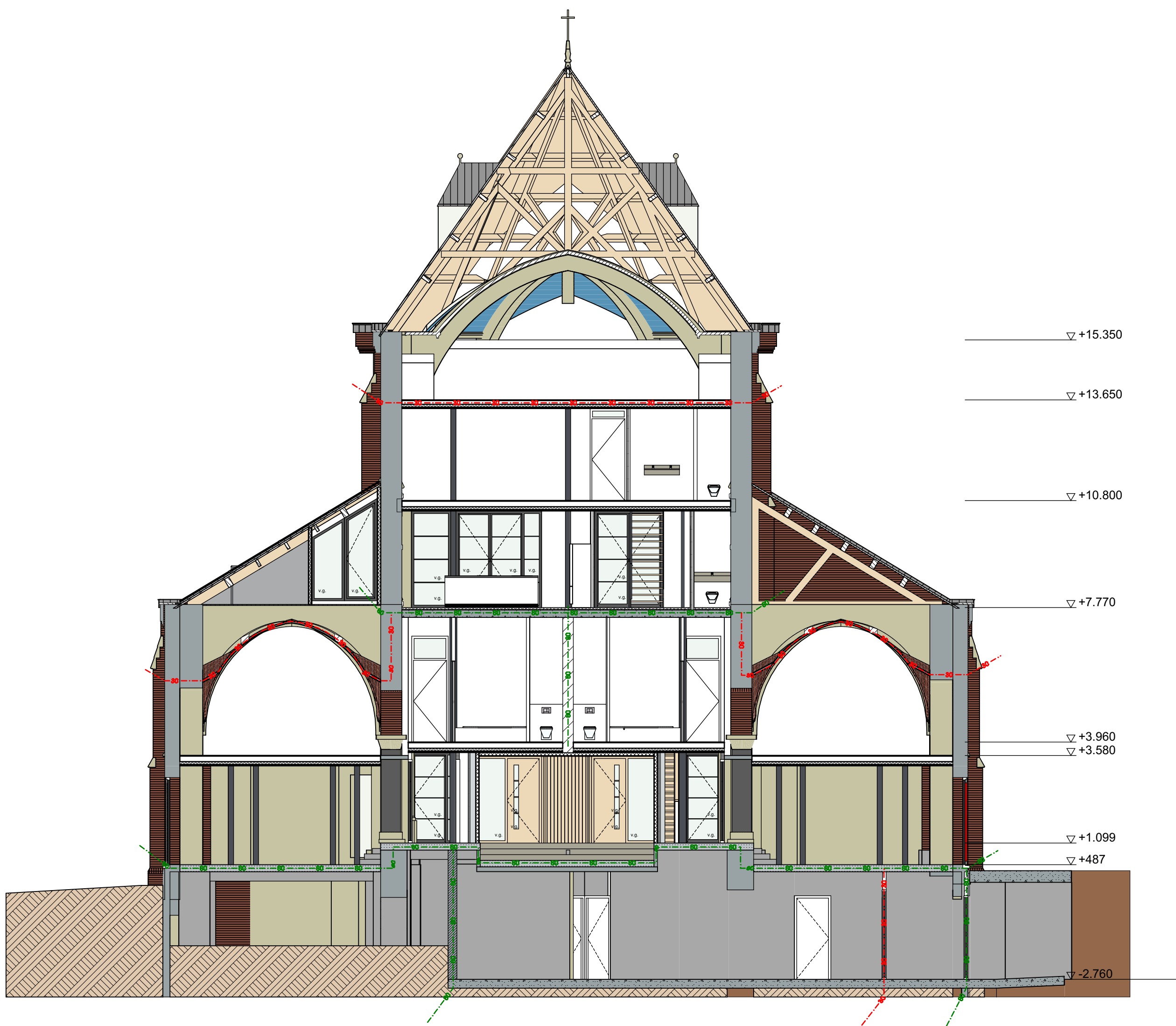
Doorsnede I-I
