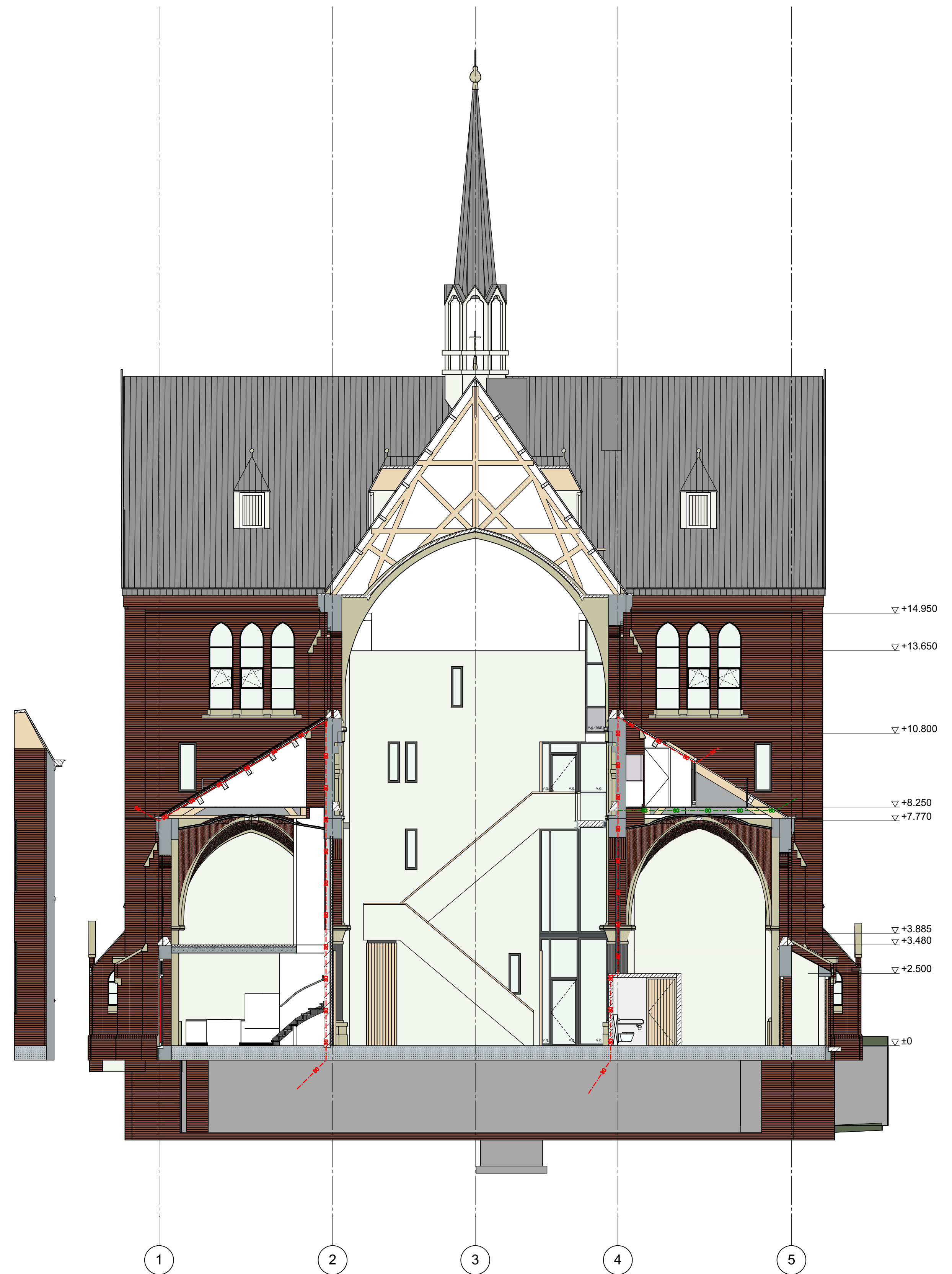
Doorsnede G-G
