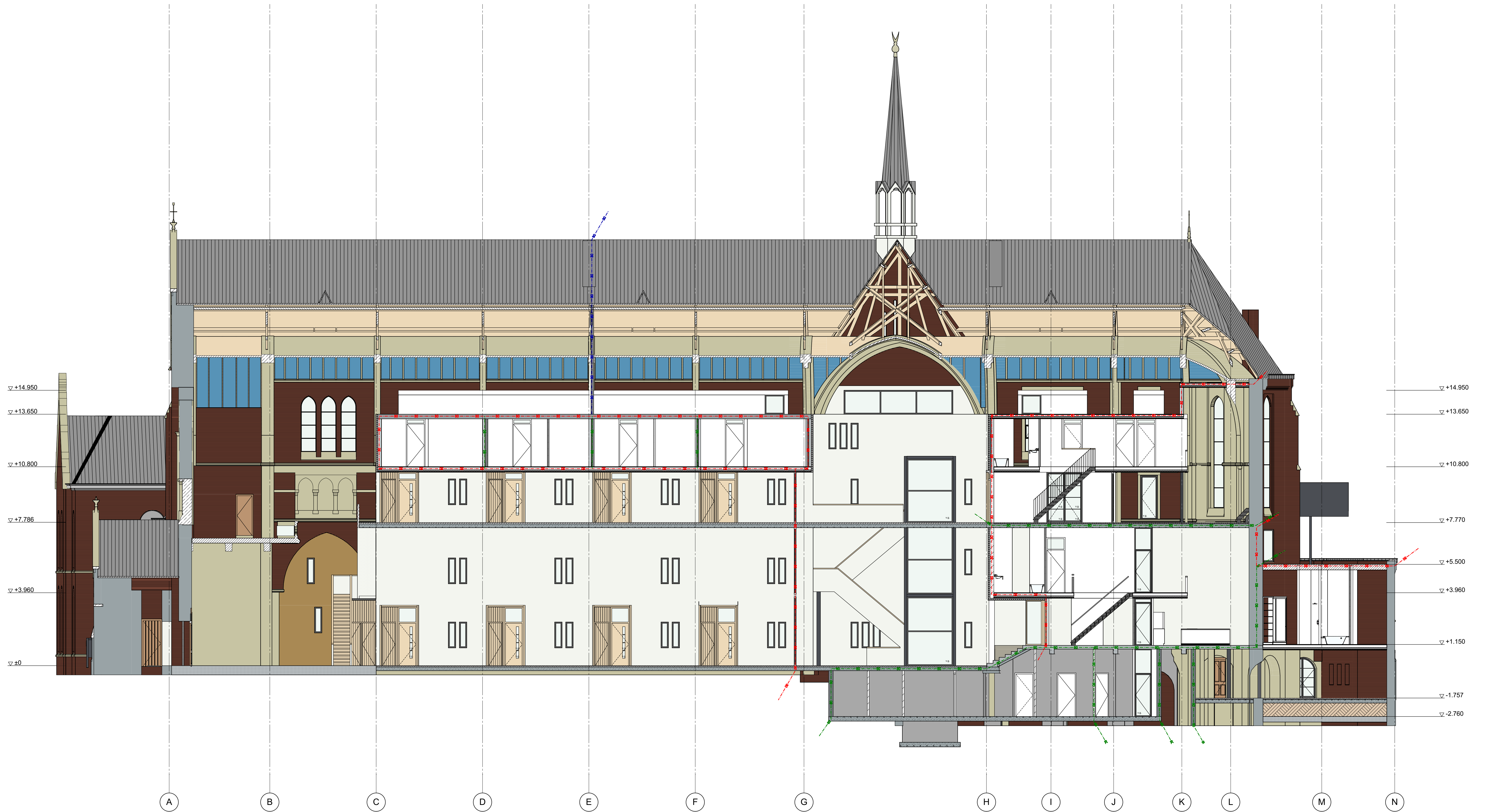
Doorsnede C-C
