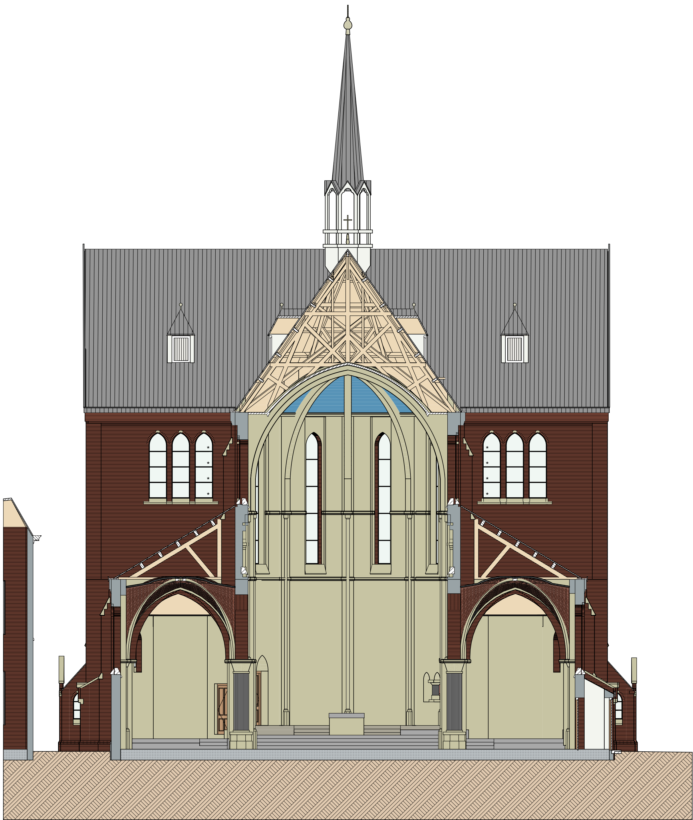
Doorsnede G-G
