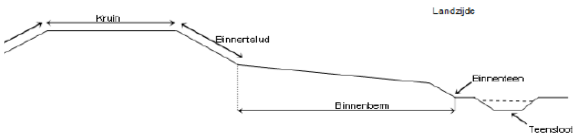
Figuur 2: Onderdelen waaruit een waterkering kan bestaan (aan polderzijde)
