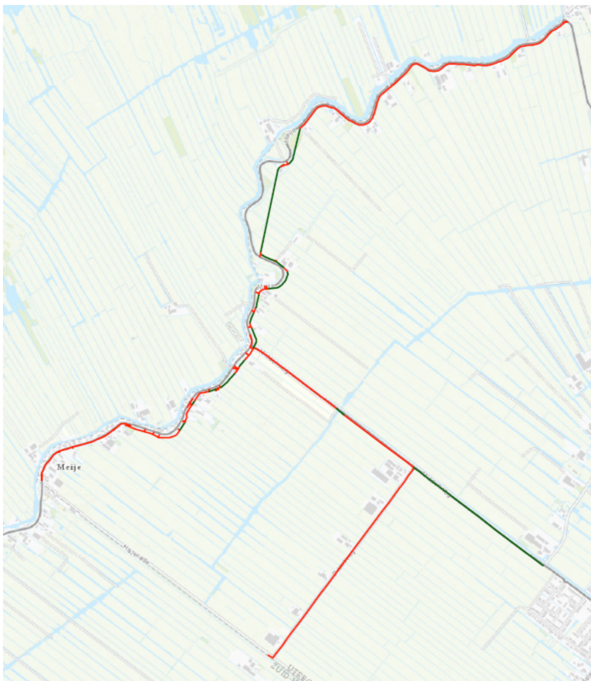
Leidingtracé met gestuurde boringen (groen) en aanleg in een sleuf (rood)
