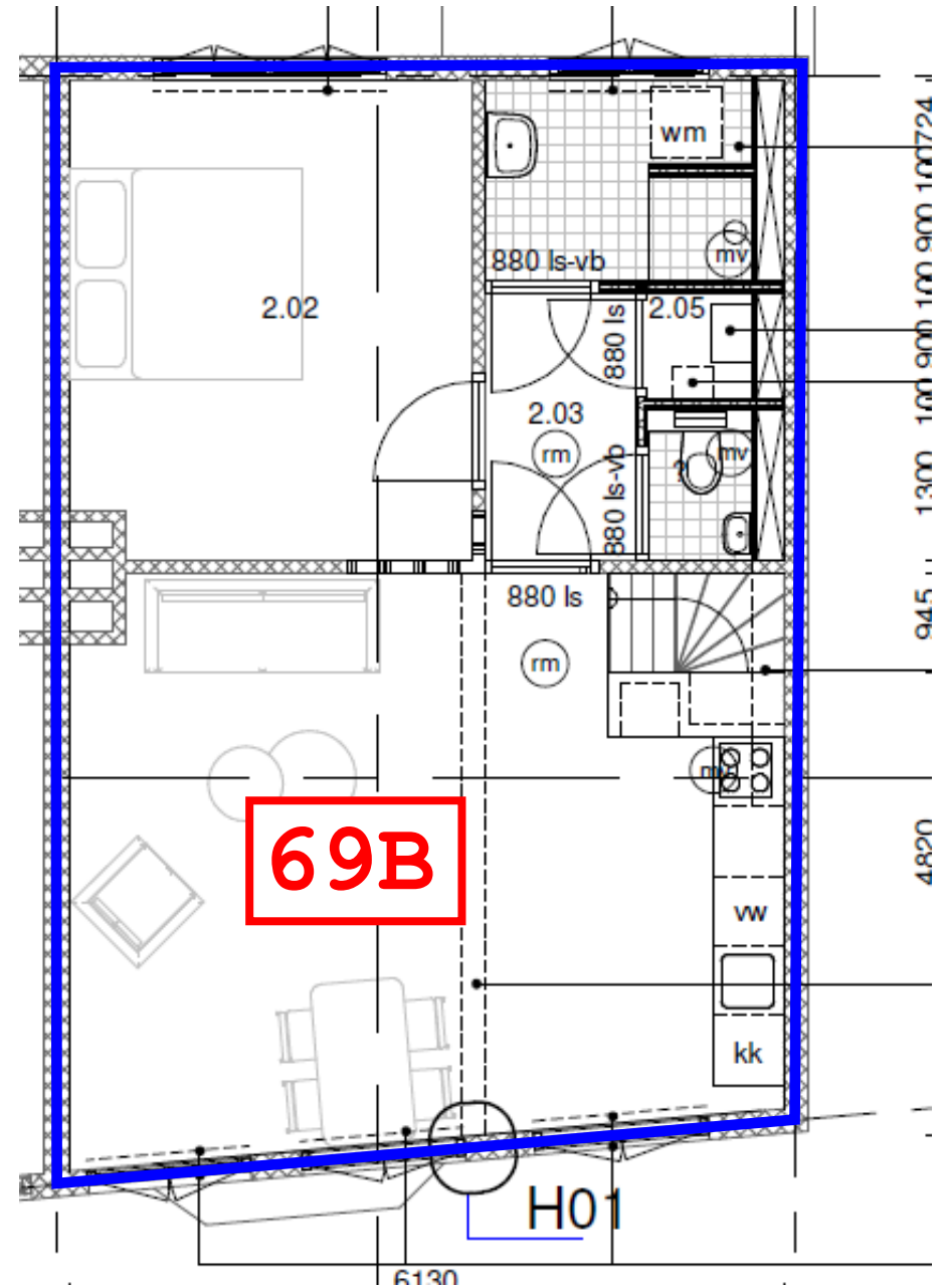
2e verdieping
