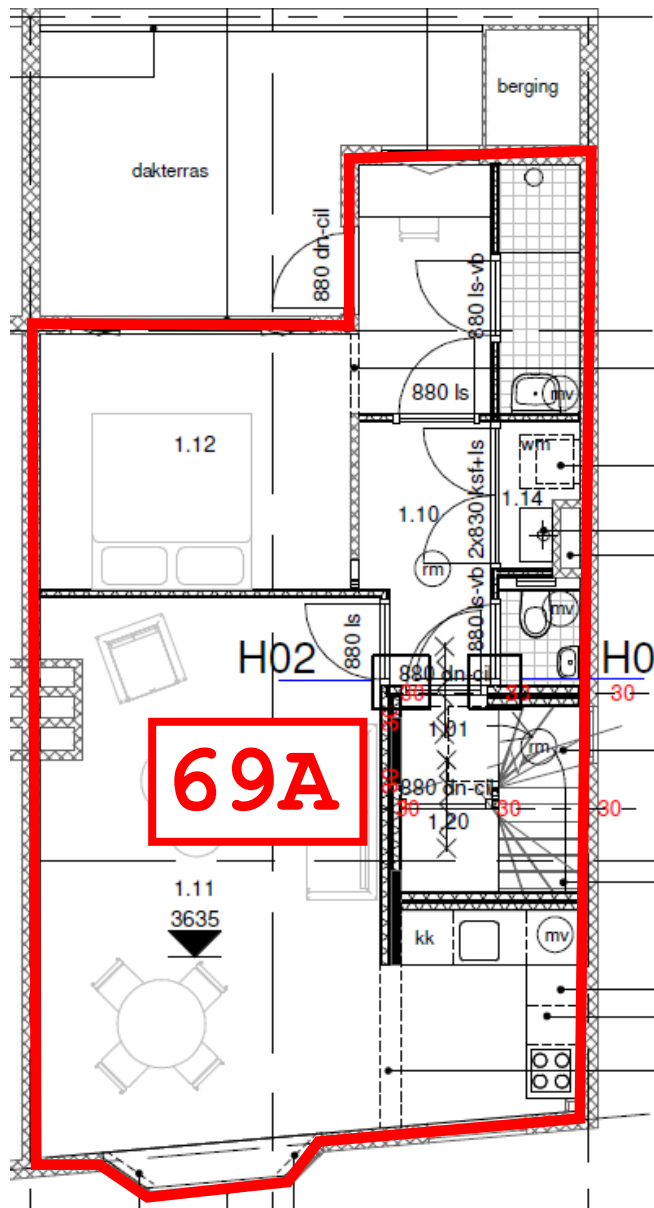
1e verdieping
