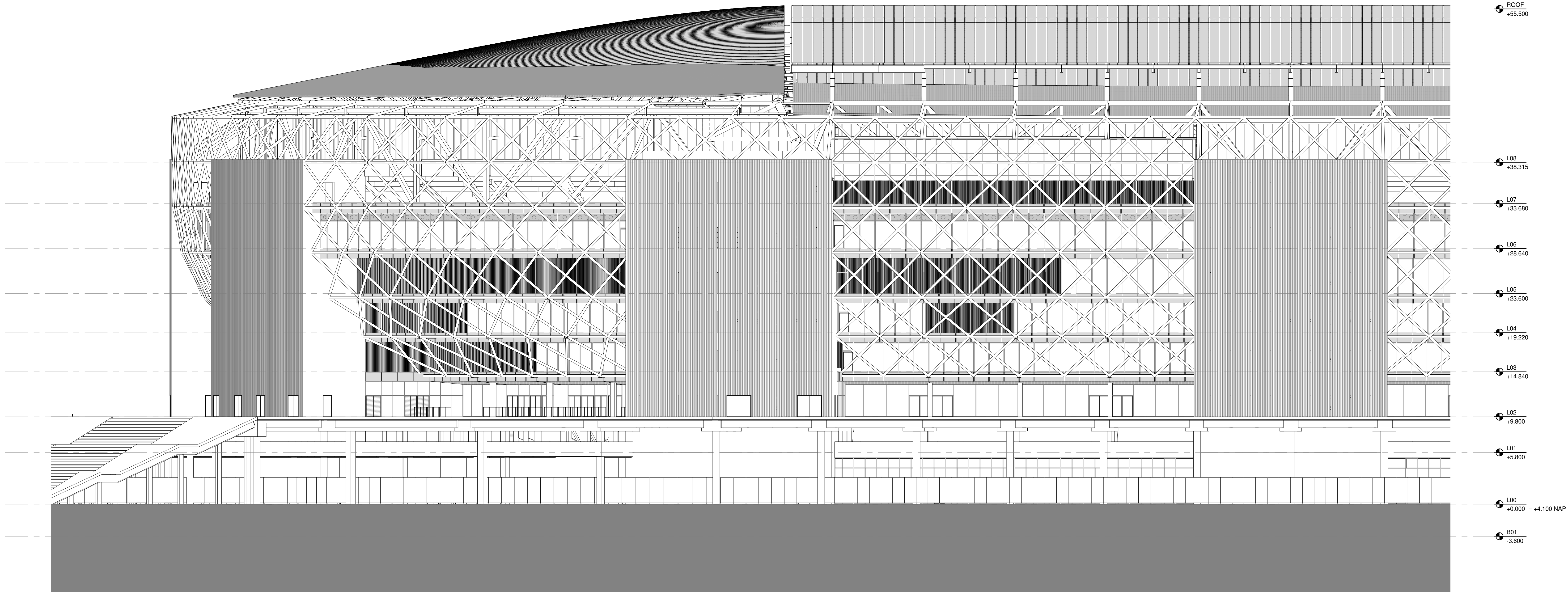
1 GEVELAANZICHT - OOST - B SCHAAAL: 1 : 200
