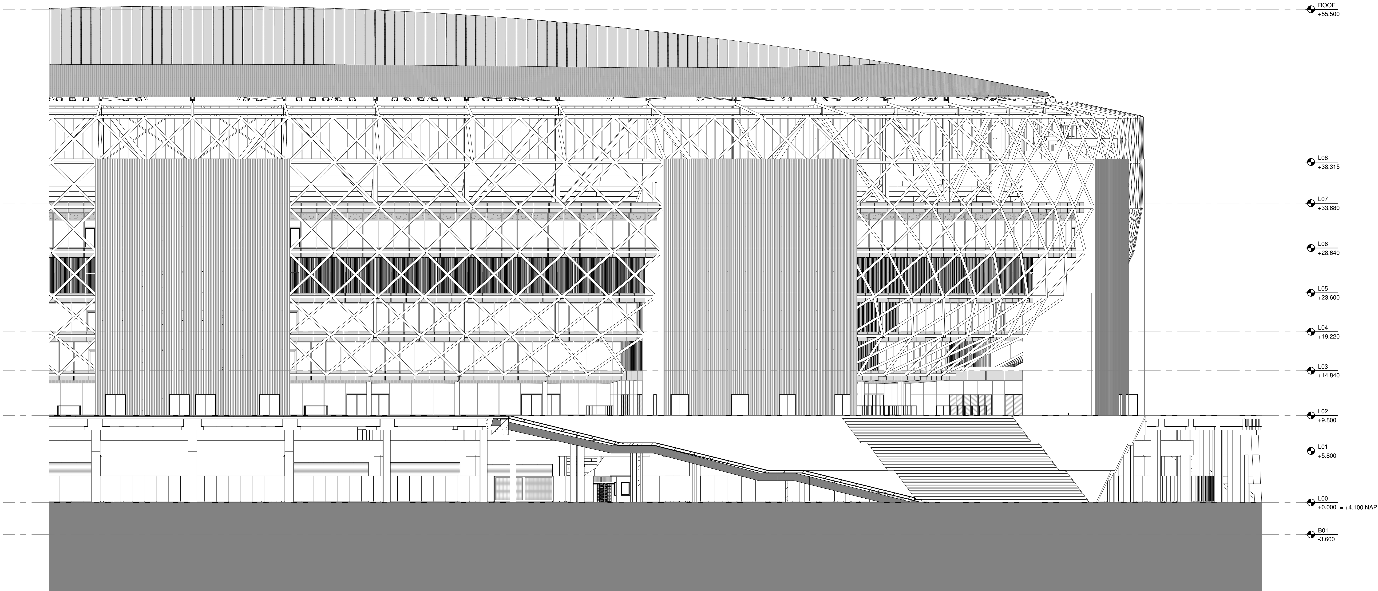
② GEVELAANZICHT - ZUID - B SCHAAAL: 1 : 200
