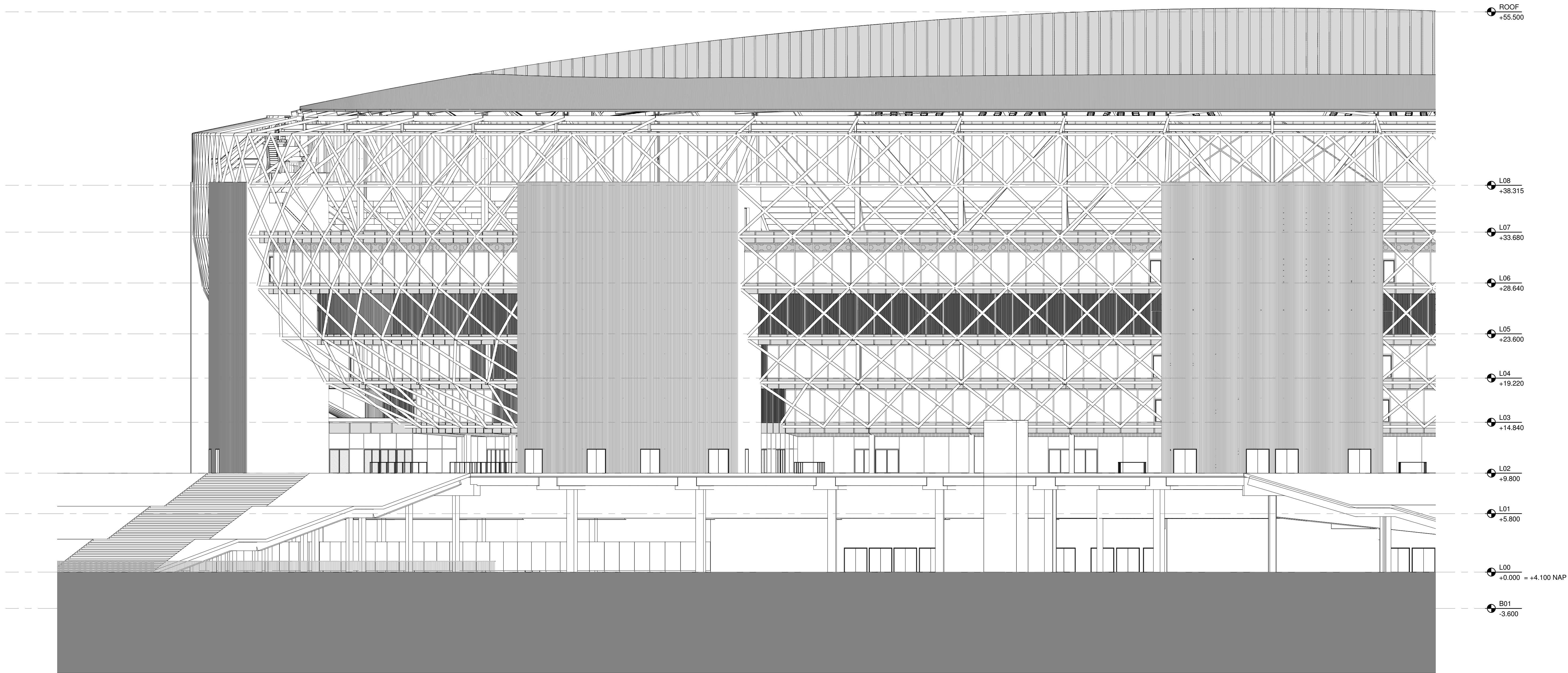
1 GEVELANZICHT - NOORD - A SCHAAL: 1 : 200
