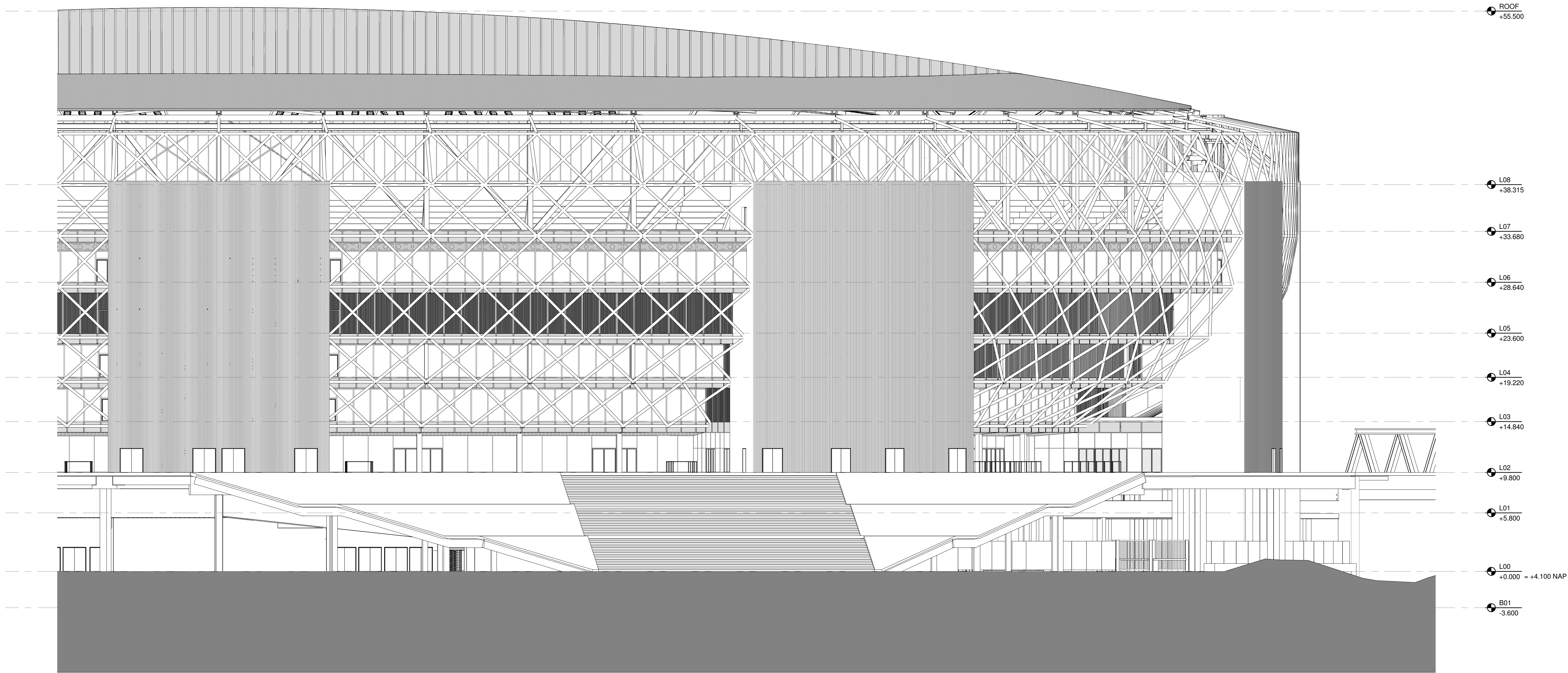
2 GEVELANZICHT - NOORD - D SCHAAL: 1 : 200
