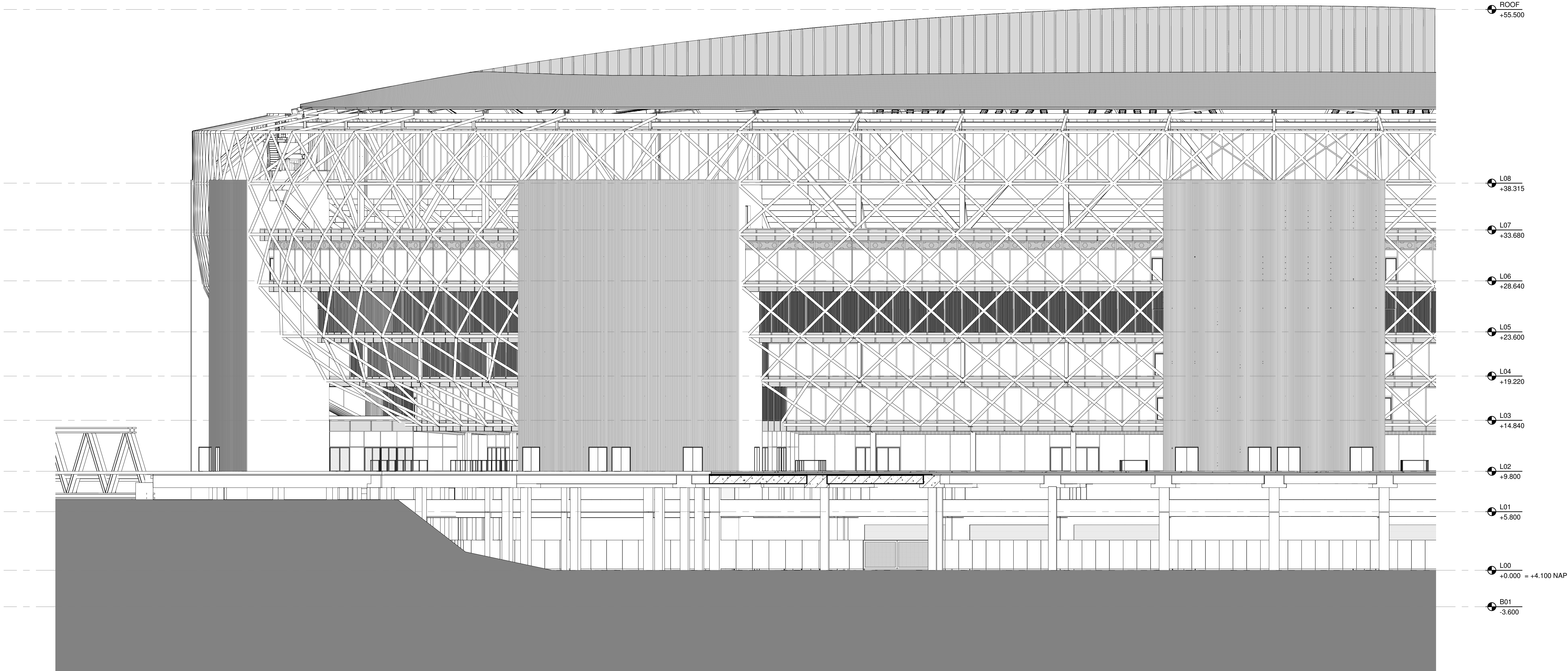
① GEVELAANZICHT - ZUID - C SCHAAAL: 1 : 200
