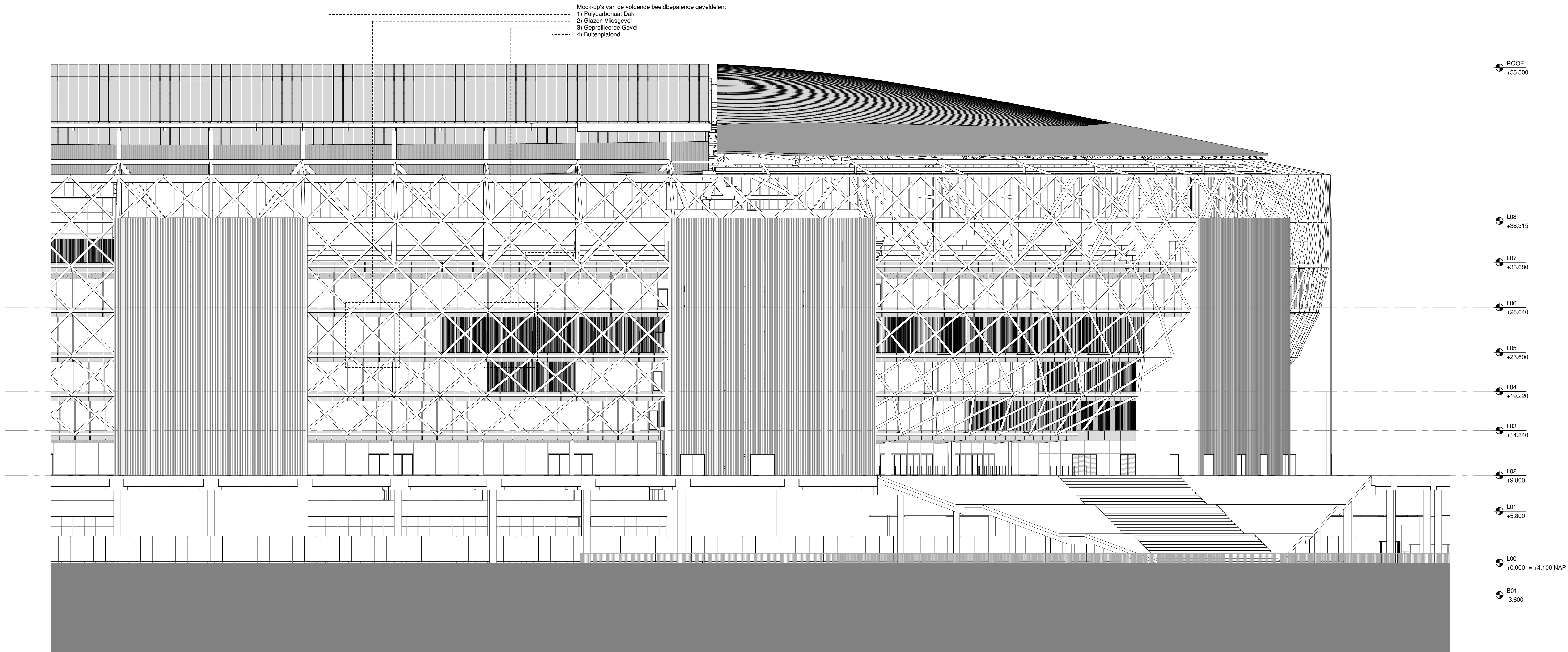
2 GEVELAANZICHT - OOST - A SCHAAAL: 1 : 200
