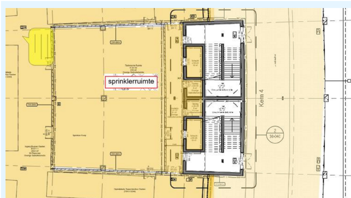
figuur 5: sprinklerpompruimte
