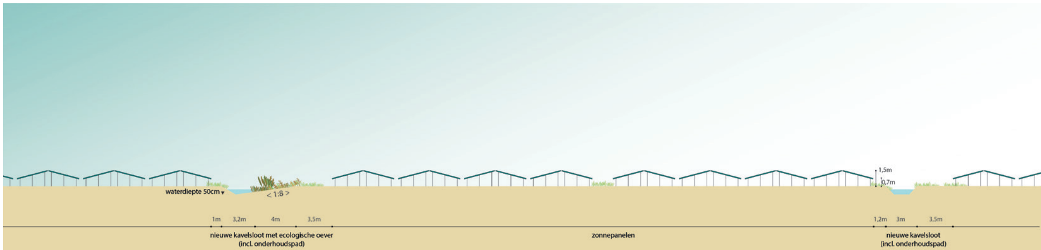
Principedoorsnede 1: nieuwe situatie, nieuwe kavelsloten waarvan één met ecologische oever, kruiden- en faunarijck grasland als onderbegroeiing.
