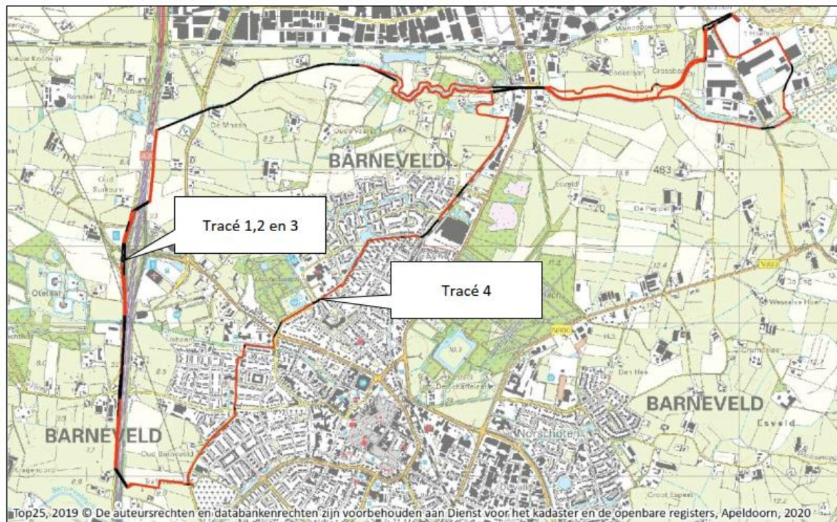
Figuur 1.1: Ligging tracés ten behoeve van de 20 kV kabelverbindingen
