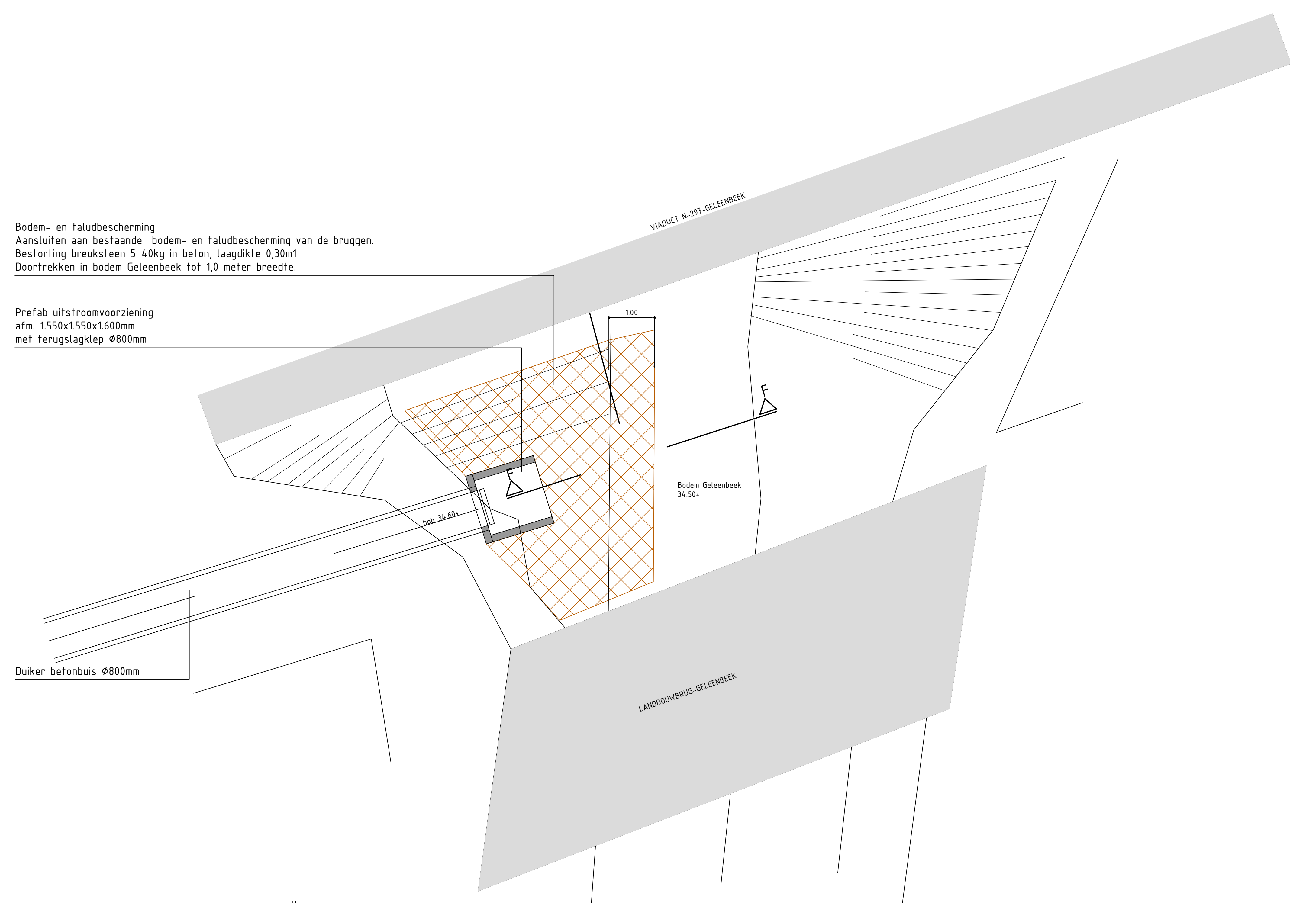
Detail 4: Situatie uitstroombak Geleenbeek Schaal 1:50
