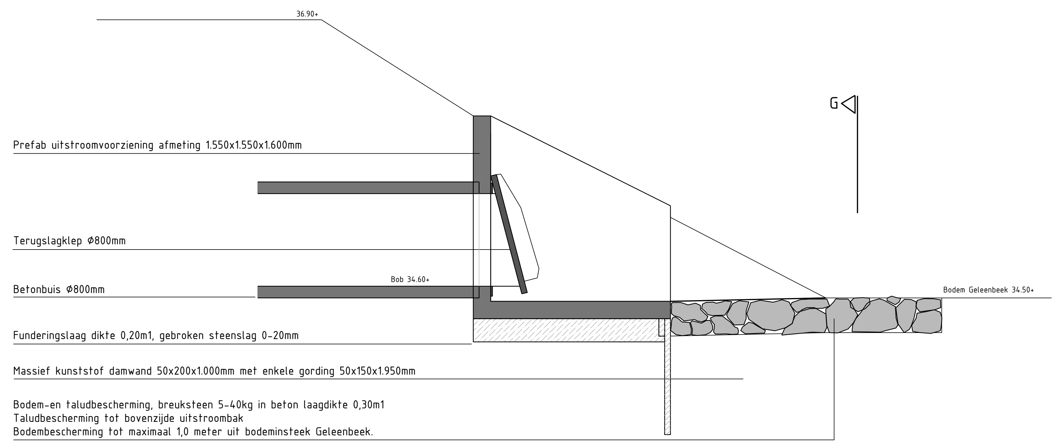
Detail 4: Doorsnede F-F uitstroombak Geleenbeek Schaal 1:20
