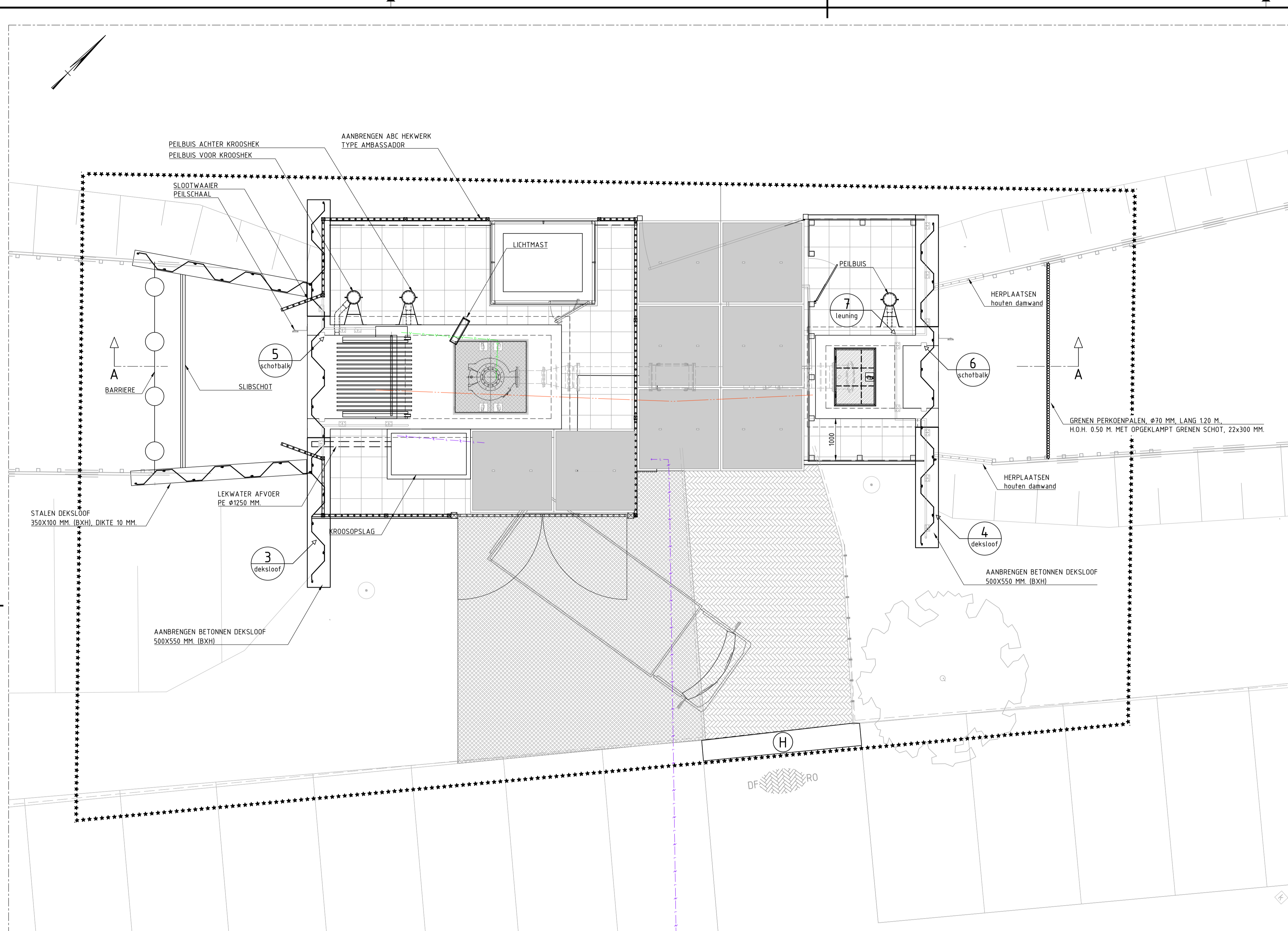
BOVENAANZICHT SCHAAL 1 : 50
