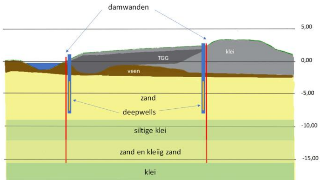
Figuur 1 doorsnede bodemopbouw en plaatsing damwanden en deepwells
