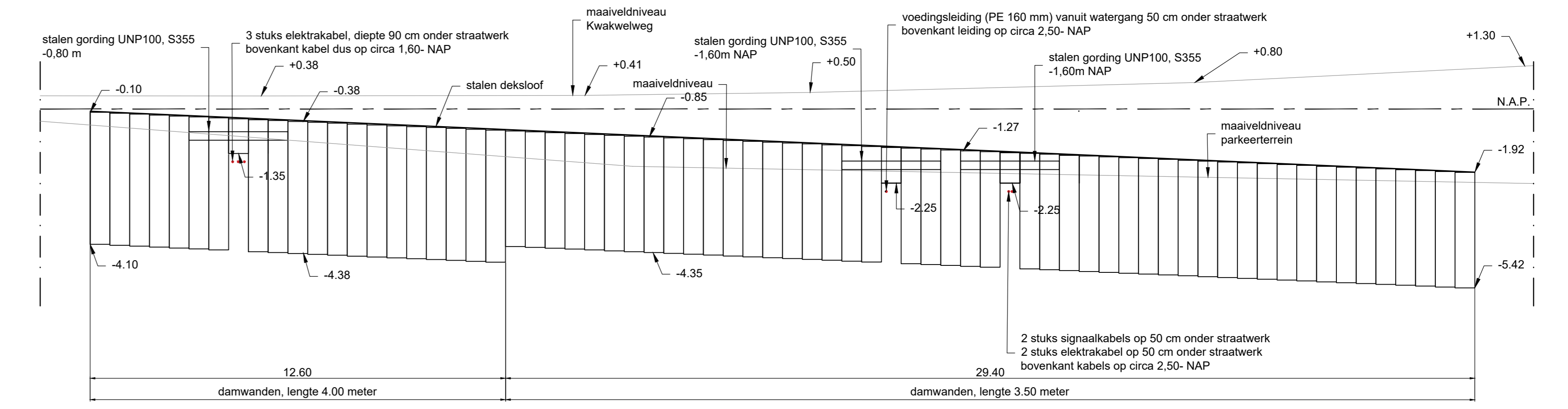
Aanzicht D-D nieuwe situatie damwandconstructie Schaal 1:100
