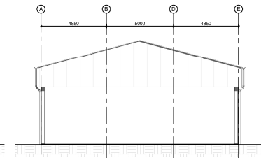
Rechter aanzicht BESTAAND
