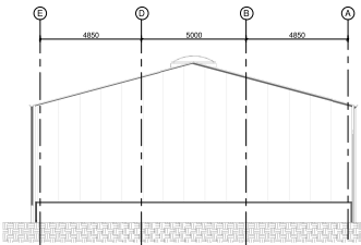
Linker aanzicht NIEUW
