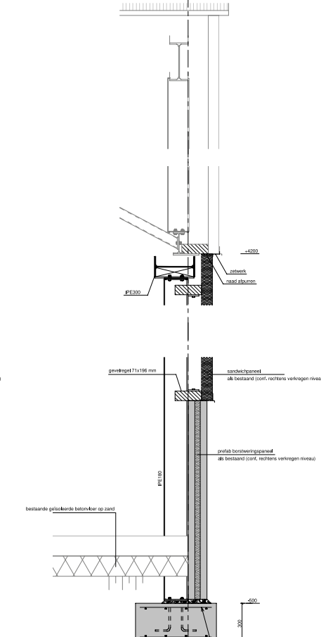
Langsdoorsnede NIEUW
