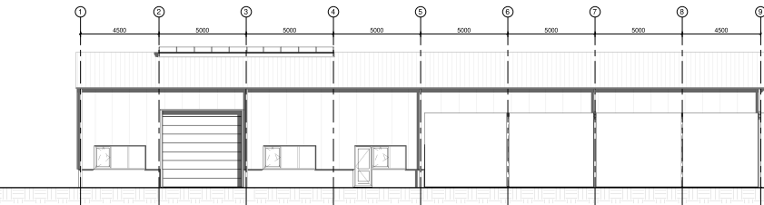
Voor aanzicht BESTAAND
