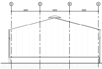
Linker aanzicht BESTAAND
