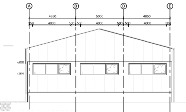
Rechter aanzicht NIEUW
