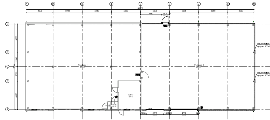
Begane Grond NIEUW
