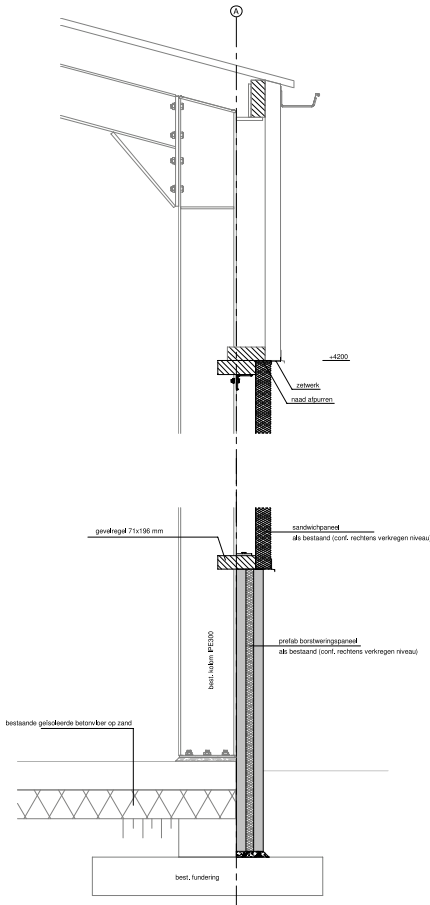
Dwarsdoorsnede NIEUW
