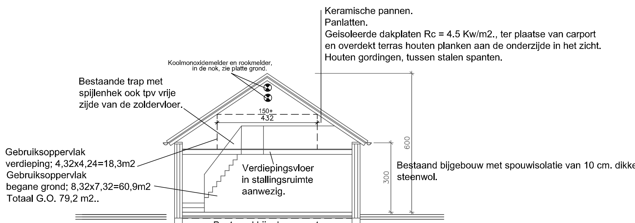
DOORSNEDE STALLINGSRUIMTE, CARPORT/MET OVERDEKT TERRAS.
