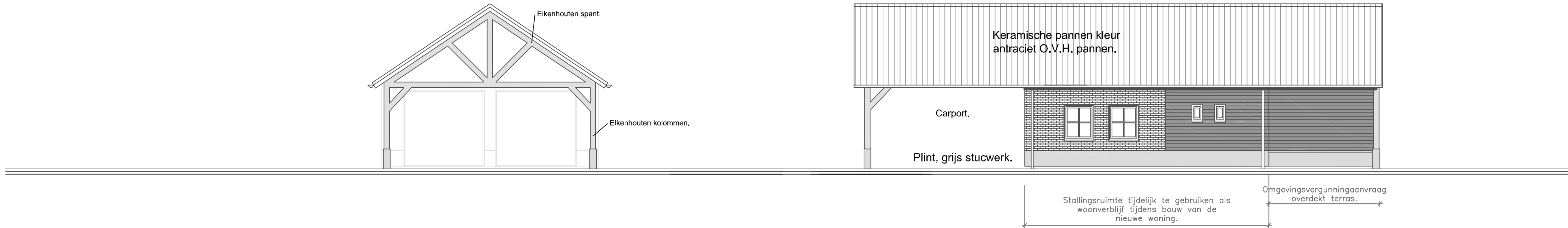
VOORGEVEL STALLINGSRUIMTE/CARPORT VANUIT VOORPEELWEG
