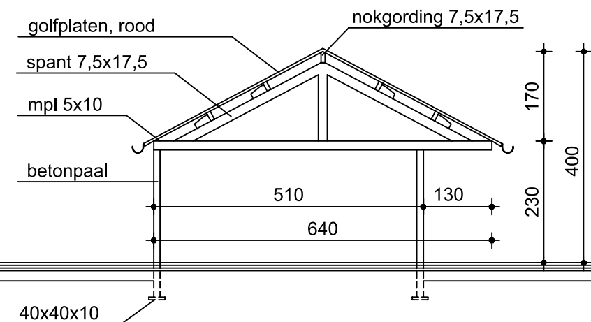
DOORSNEDE
