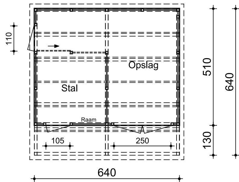
PLATTEGROND
