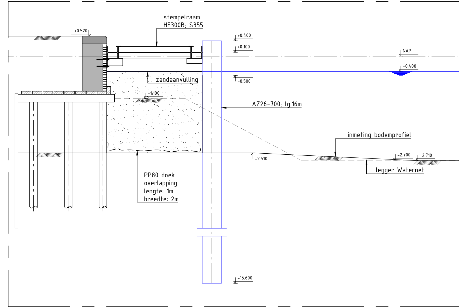
DOORSNED C-C SCHAAL 1:50
