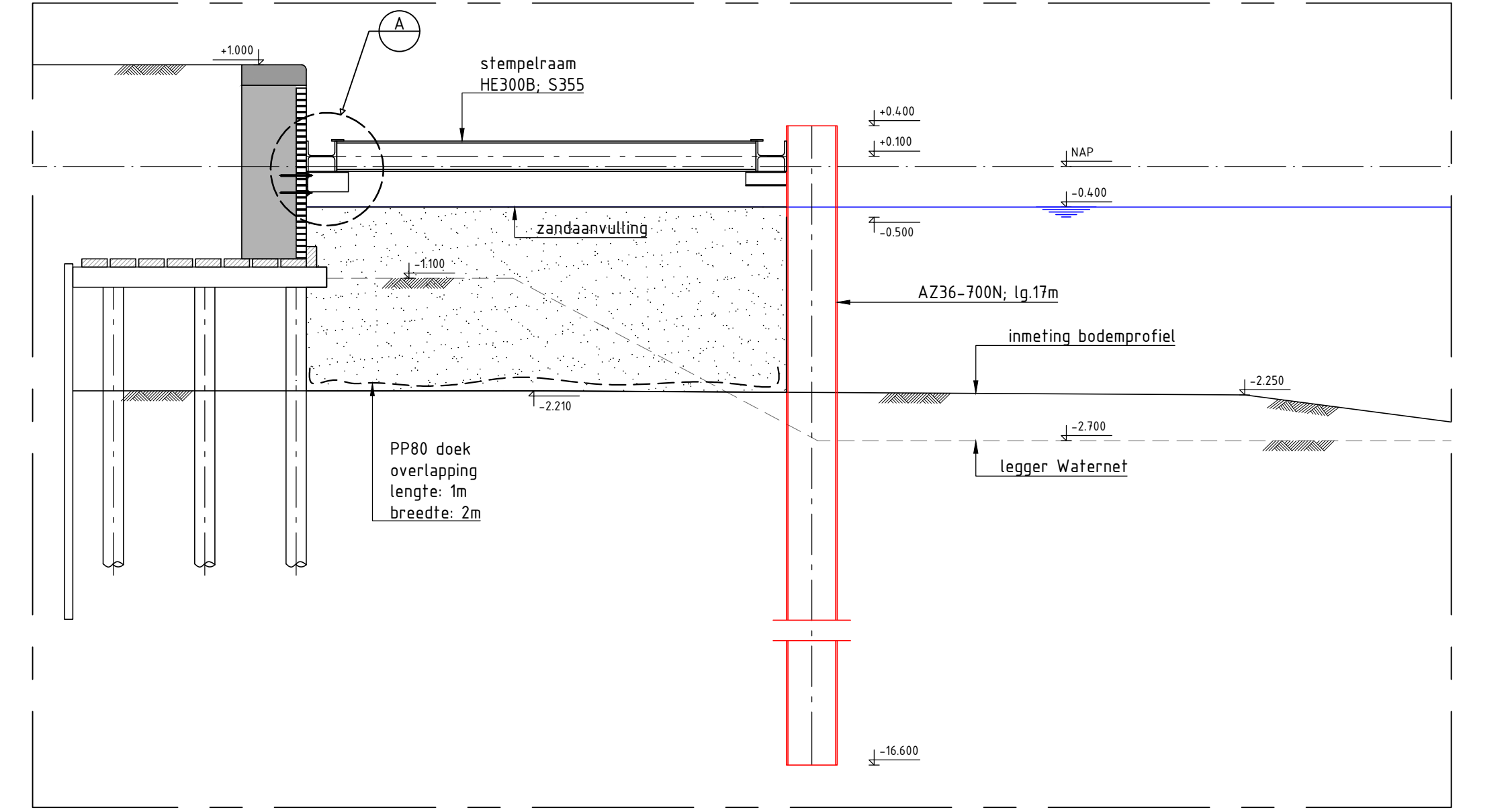
DOORSNED A-A SCHAAL 1:50
