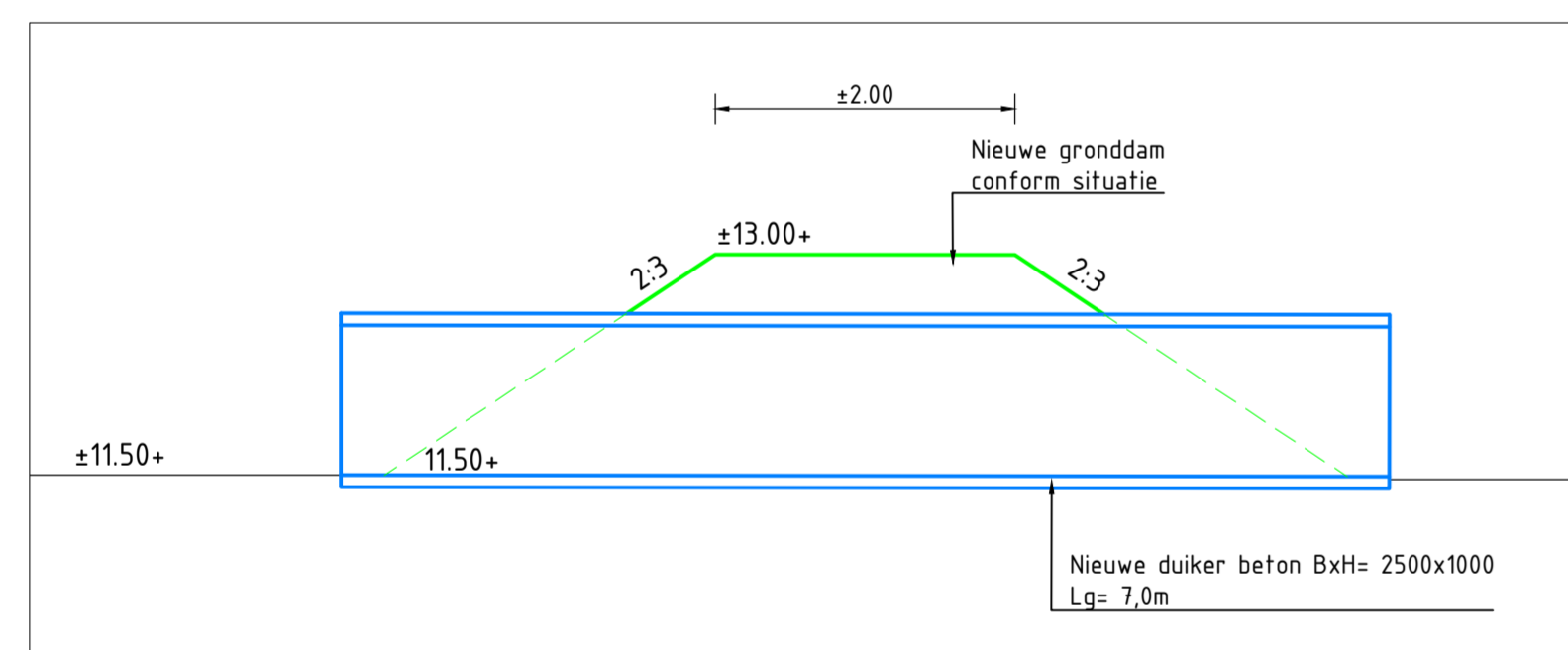
Doorsnede diiker 10 in gronddam Schaal 1:50
