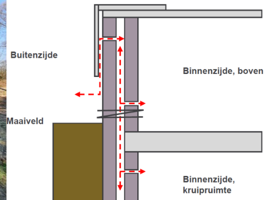
Figuur 3: Trafohuisje waar kelder en bovenbouw voor vlemuizen worden/ zijn ingericht, rechts dwarsdoorsnede.
