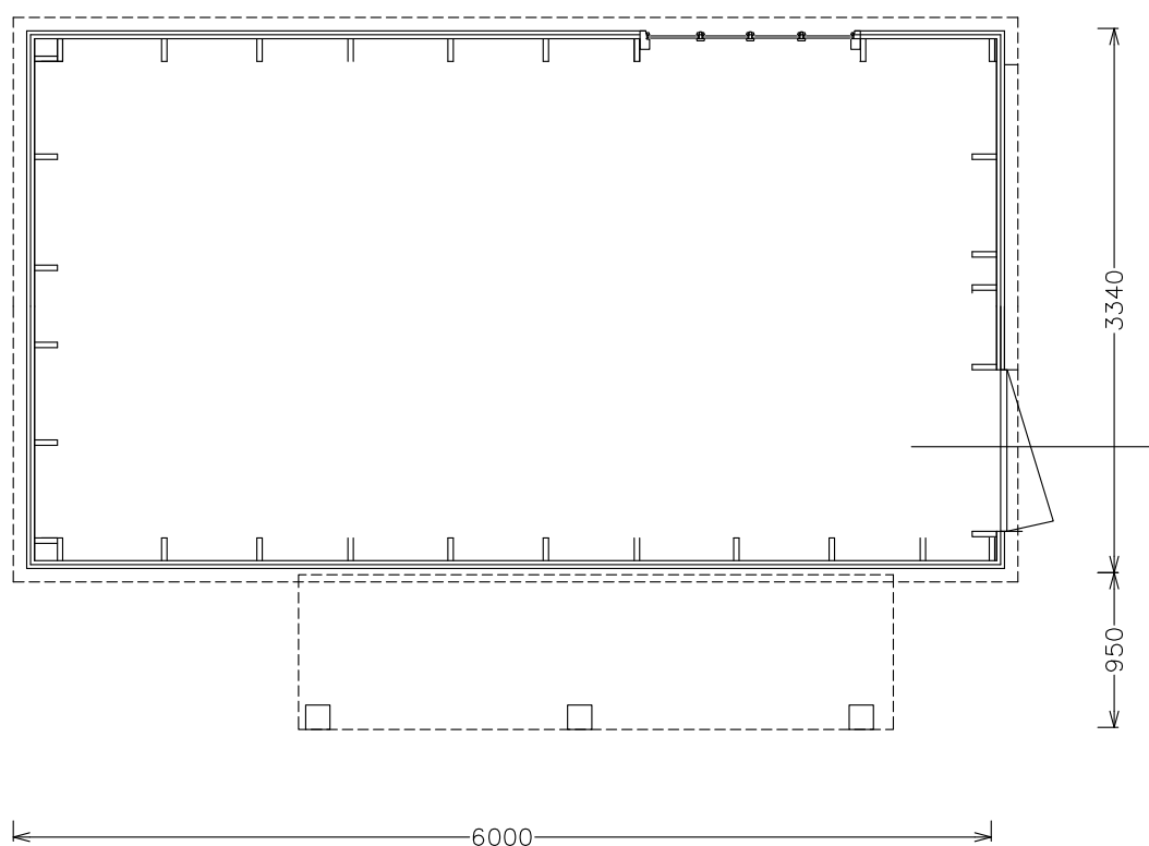
plattegrond schuur
