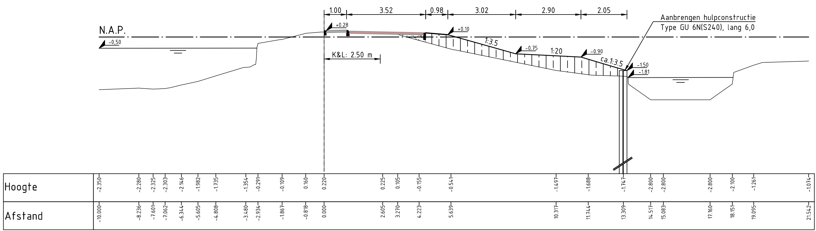
DWARSPROFIEL 6B.0ost DP1 Schaal 1:100
