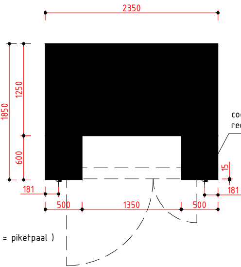
FUNDERING GESTABILISEERD ZAND dikte volgens opgave constructeur
