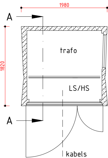
PLATTEGROND
