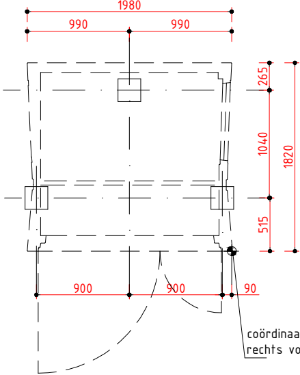
PALENPLAN
