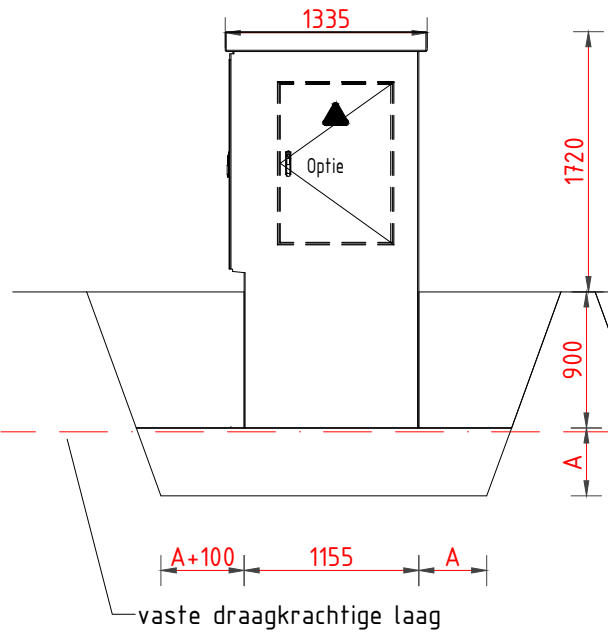
RECHTERZIJAANZICHT
