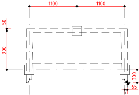
PALENPLAN
