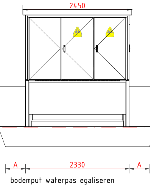
VOORAANZICHT
