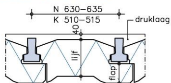
DOORSNEDEN ISOLATIEVLOER
