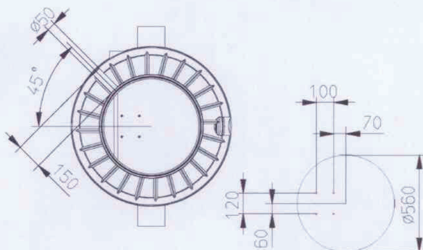
BODEMPLAAT
