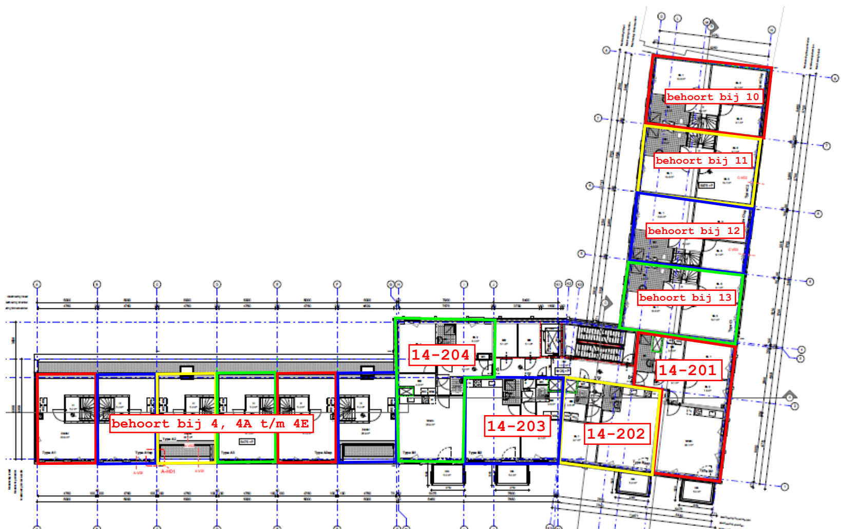
2e verdieping
