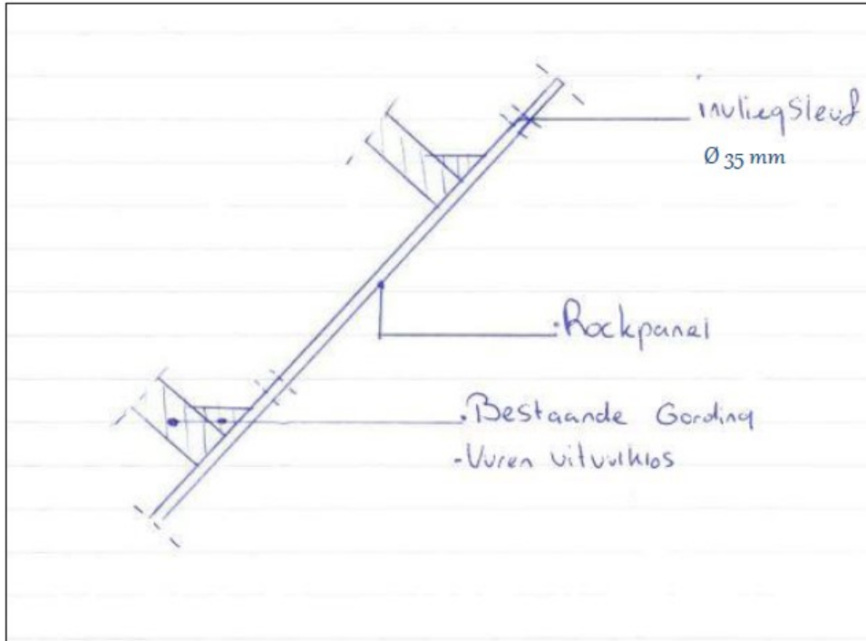
Figuur 3. Nestplaats voor huismus in overstek boven de gording (6 nestplaatsen per kopgevel).
