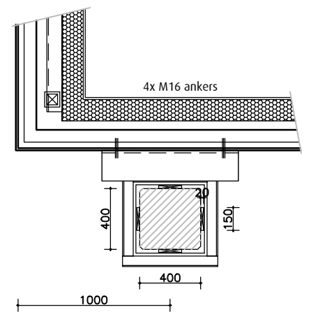
Bovenaanzicht afmeerbeugel
