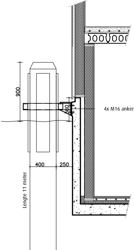
Zijaanzicht afmeerbeugel
