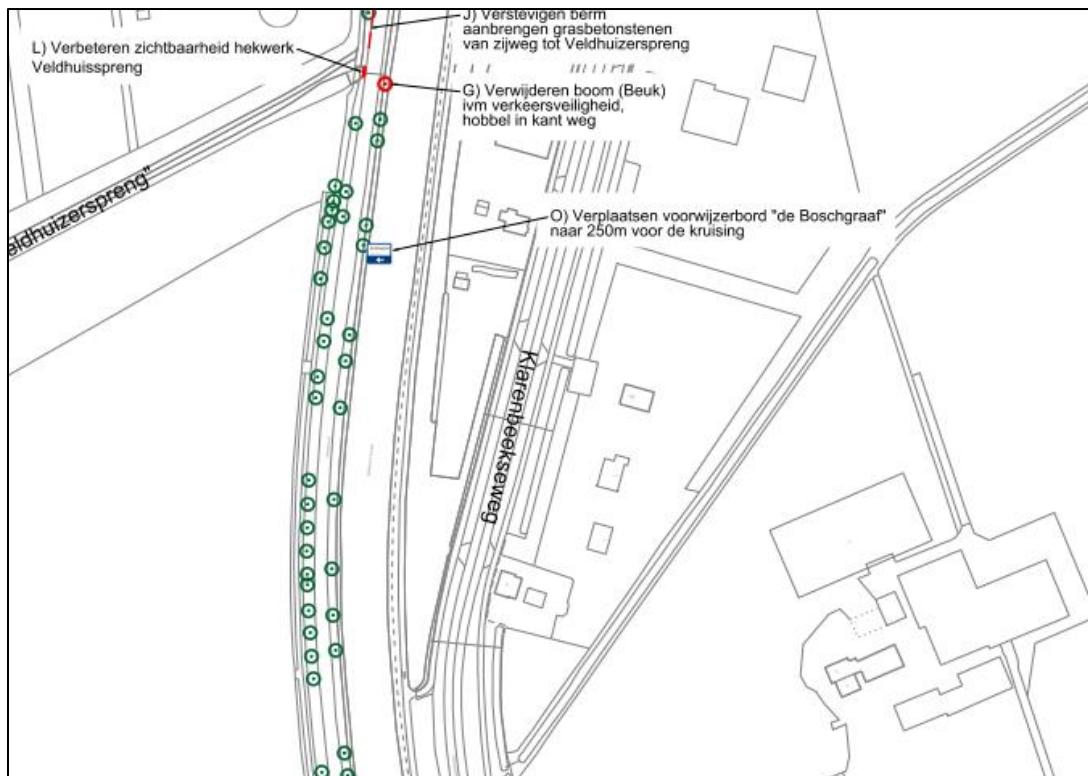
Situatietekening 3
