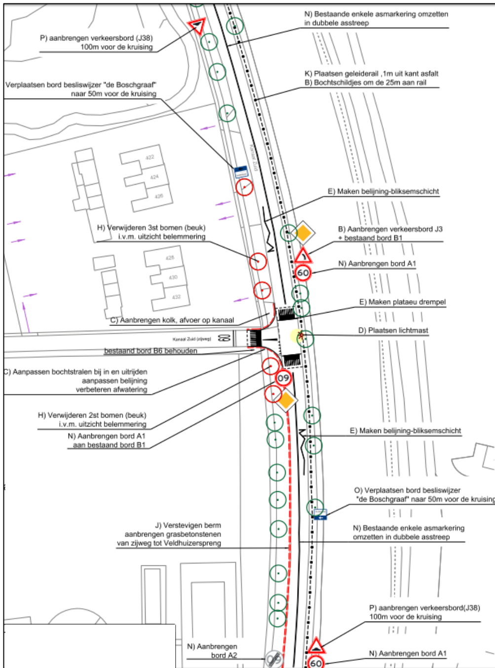
Situatietekening 2
