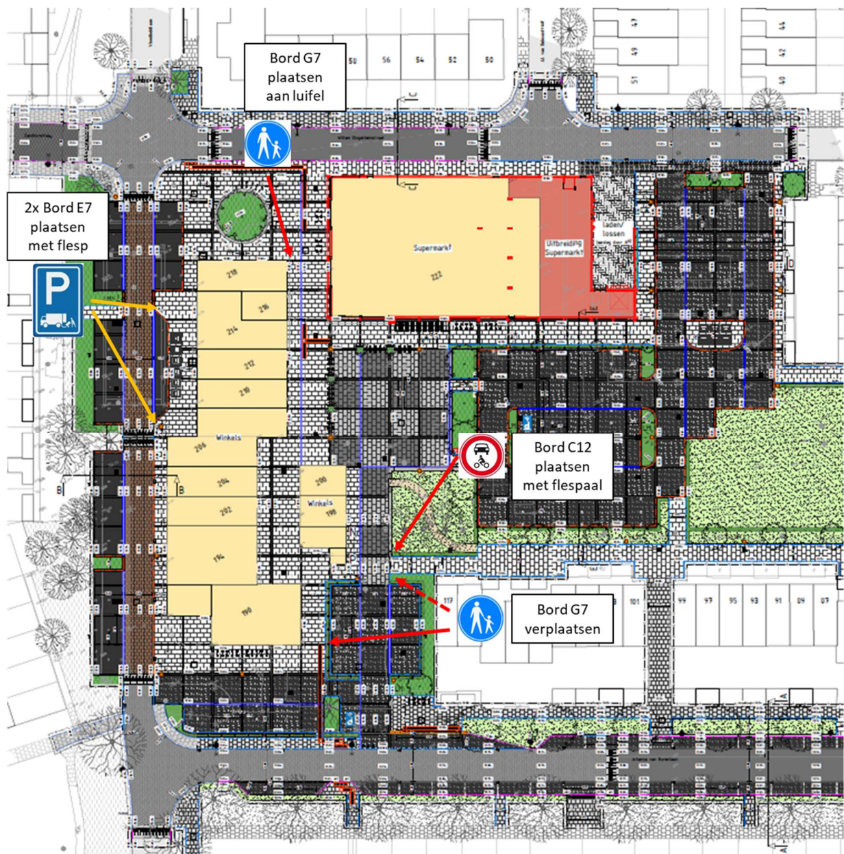
Figuur 1: Overzicht nieuwe bebording WKC De Thij
