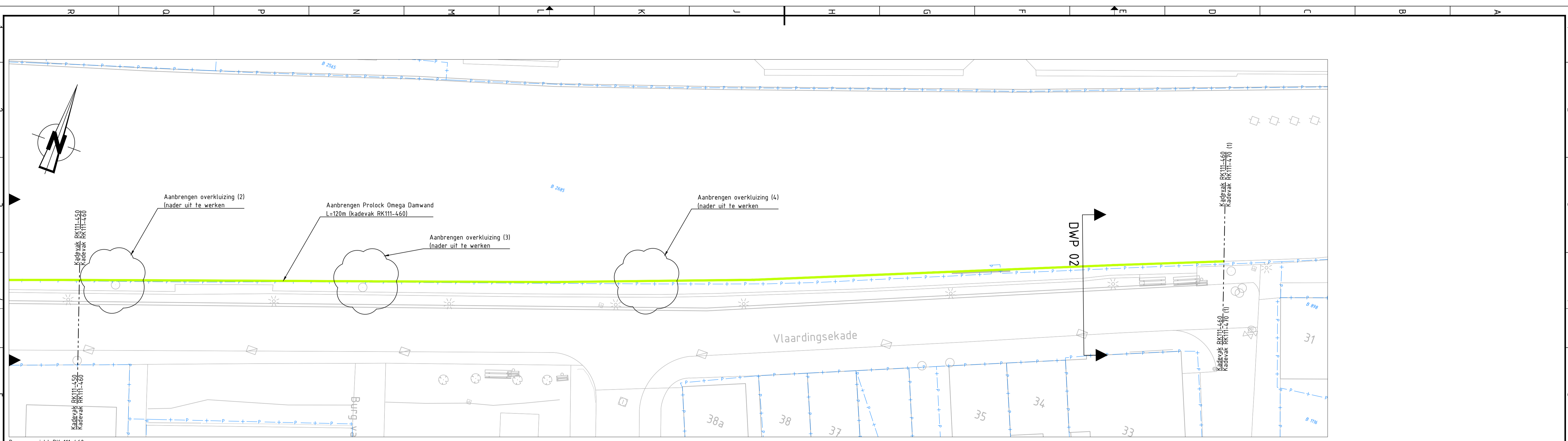
Bovenaanzicht RK 111-460 1:200
