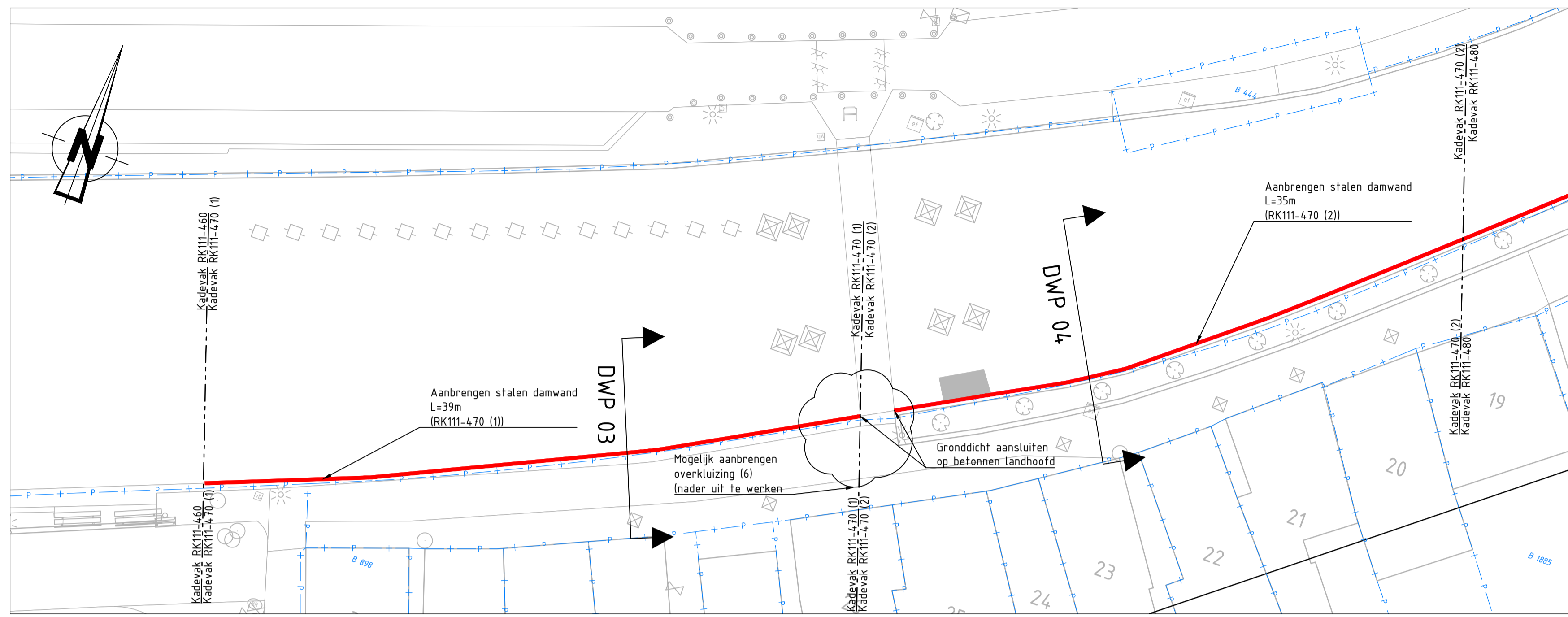
Bovenaanzicht RK 111-470 (1+2) 1:200
