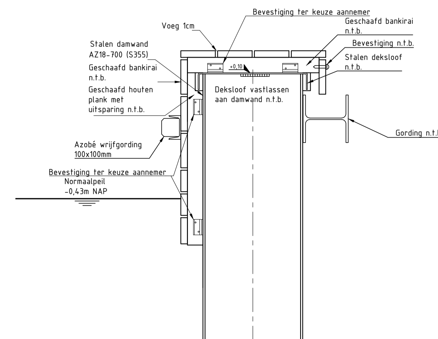
Detail stalen damwand met houten voorhangschoot en houten deksloof Kadevak RK111-470 (1) + RK111-470 (2) Schaal 1:10
