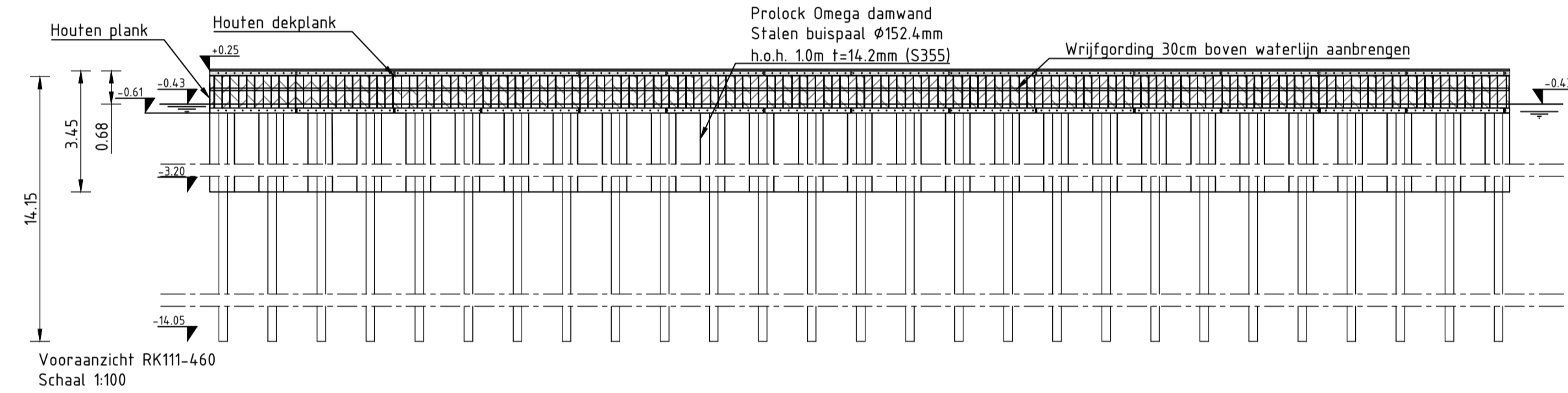
Vooranzicht RK111-460 Schaal 1:100
