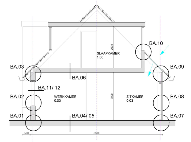
Overzicht details doorsnede
