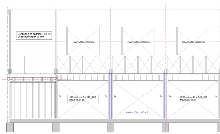
Wandaanzicht G
