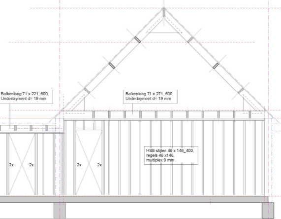
Wandaanzicht D
