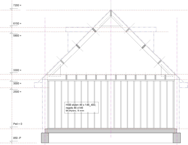
Wandaanzicht A
