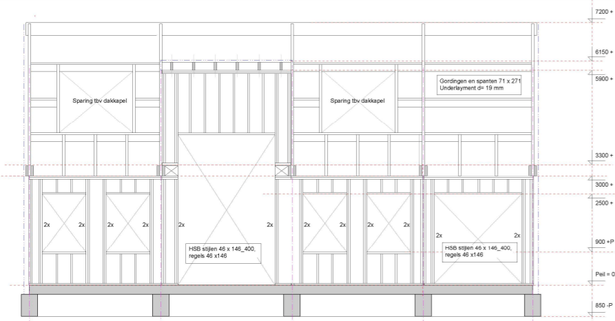
Wandaanzicht F
