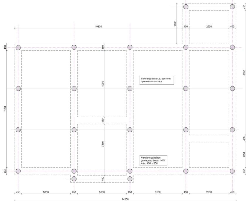
Palenplan
