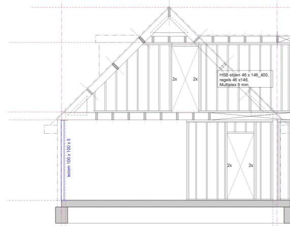
Wandaanzicht C
