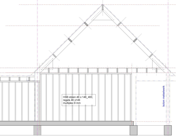
Wandaanzicht E
