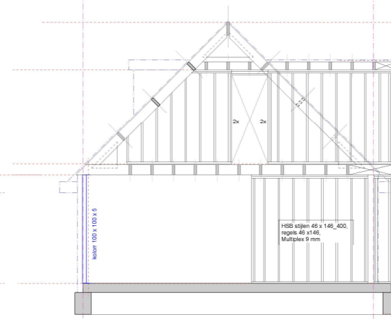
Wandaanzicht B
