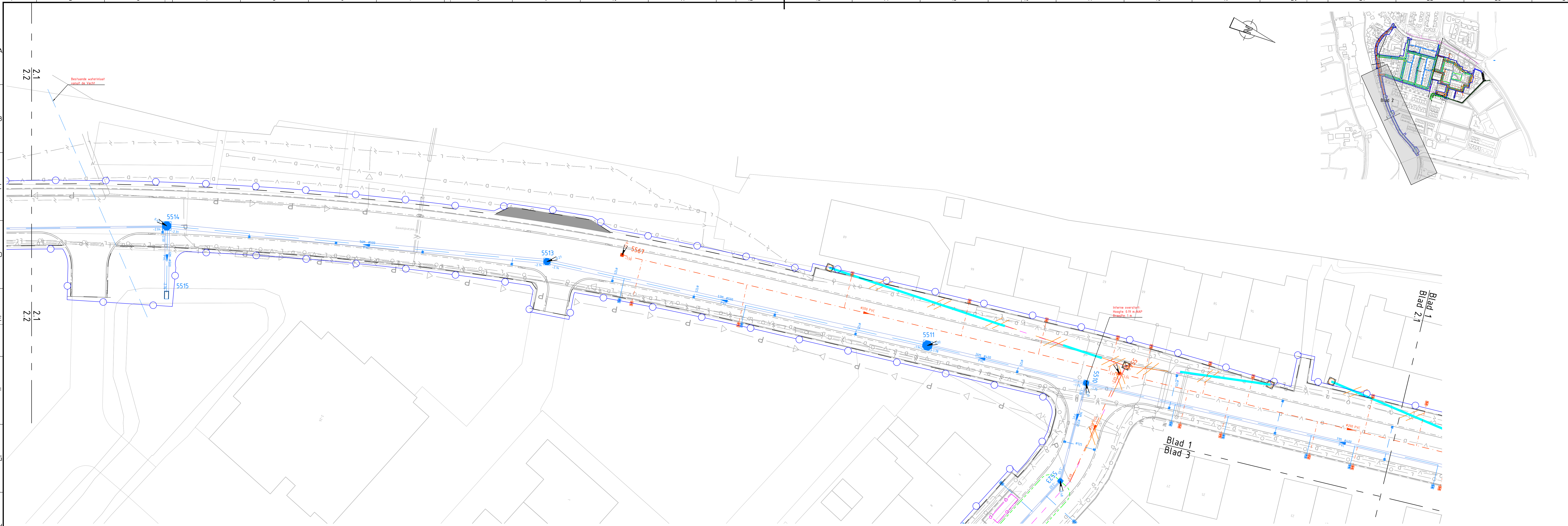
SITUATIE SCHAAL 1 : 200
