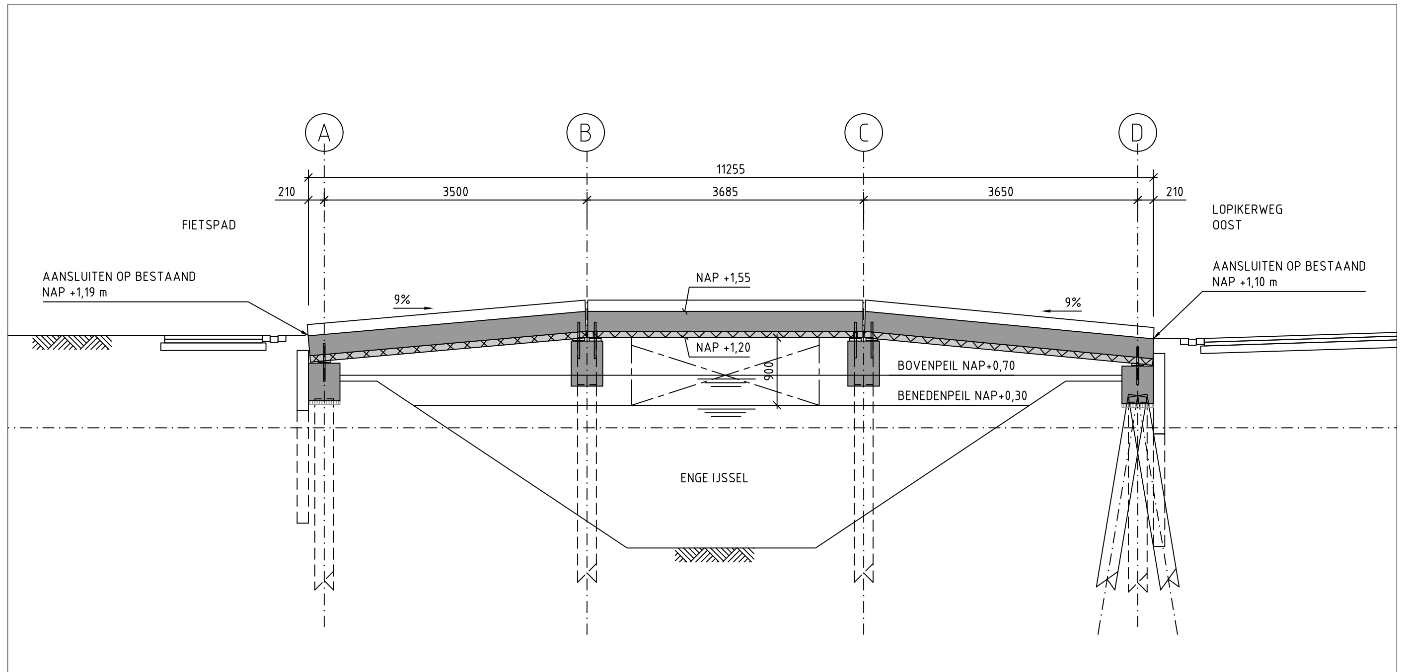
Hoogtemaatvoering Scholmanbrug
