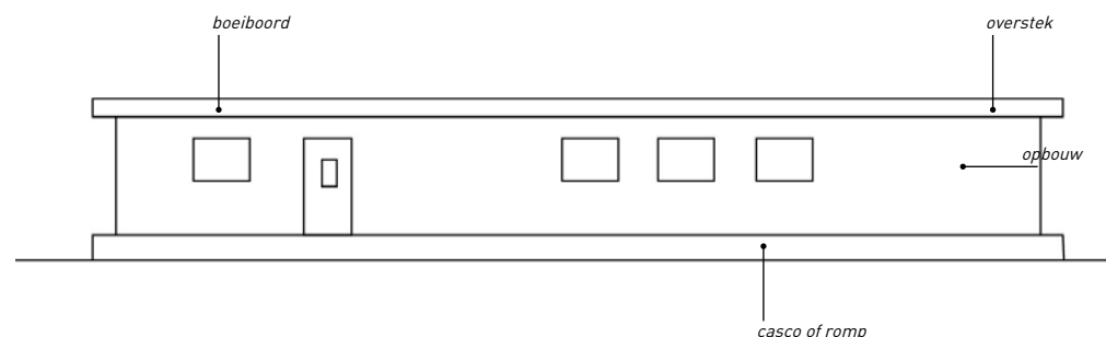
woonark
