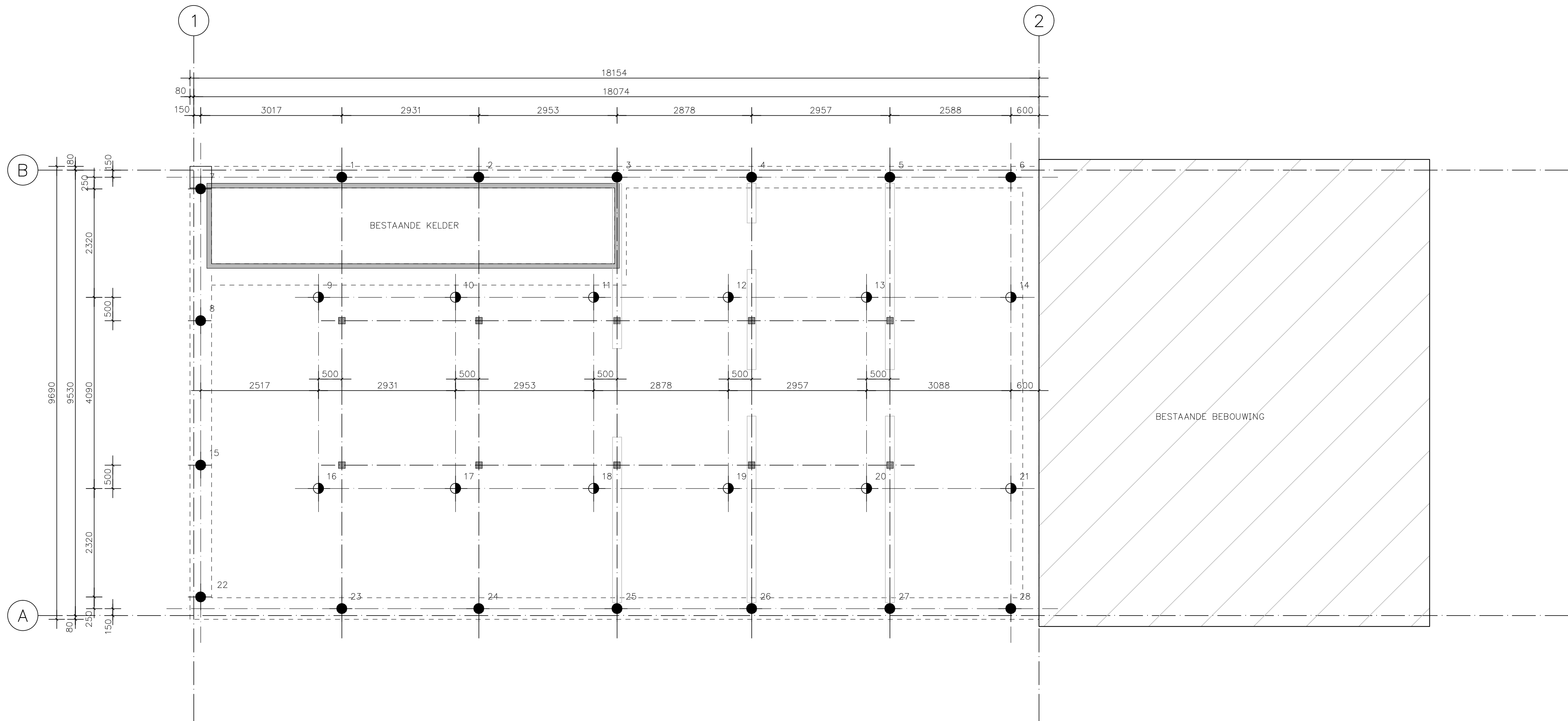
PALENPLAN.
