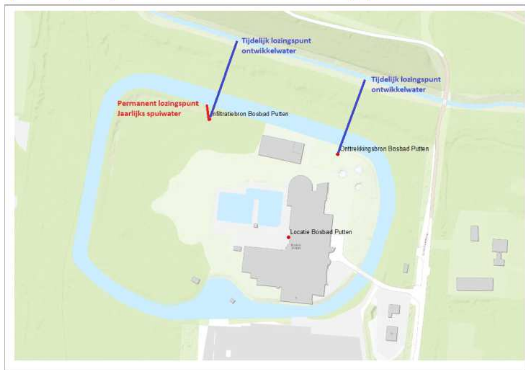
Figuur 4.2: lozingsroute spui- en ontwikkelwater ten behoeve van het bodemenergiesysteem van het Bosbad
