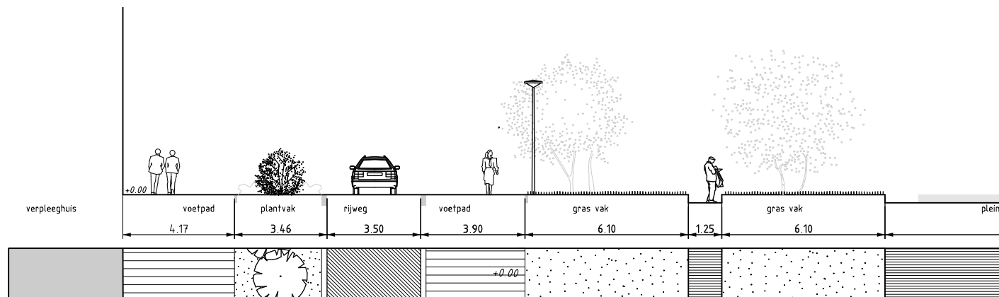
Profiel A
