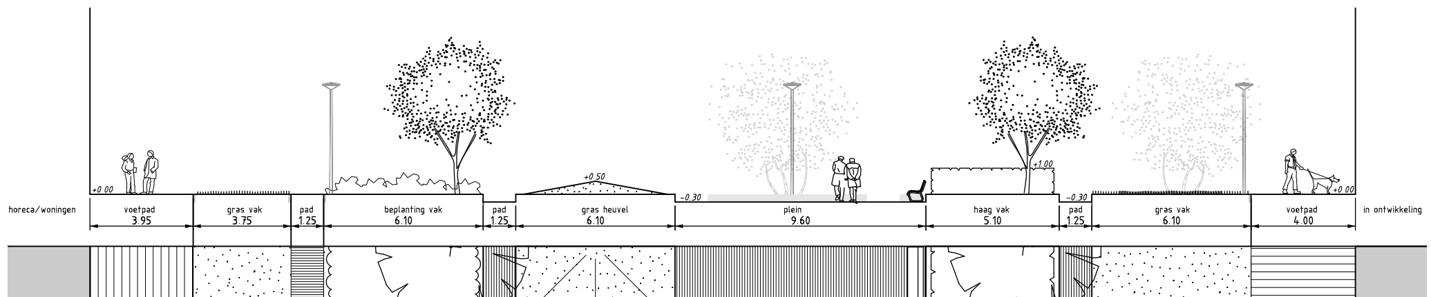
Profiel C
